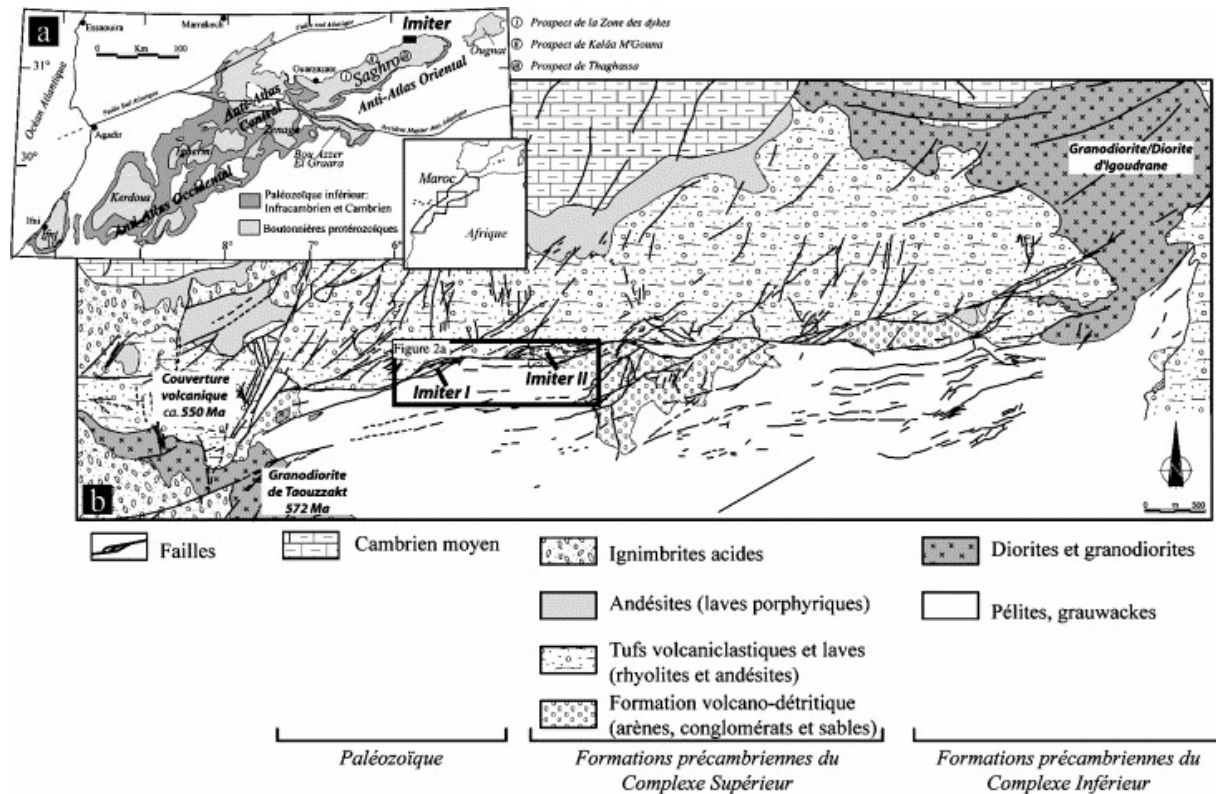
Fig. 1. (a) Représentation schématique de l'Anti-Atlas marocain et localisation de la mine d'Imiter et des autres indices minéralisés du Jbel Saghro. (b) Carte géologique simplifiée du gisement d'Imiter (d'après documents SMI).
