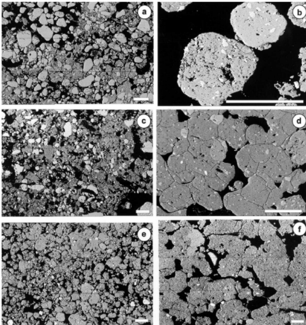
Figure 1. Mode d'assemblage des microagrégats observés en microscopie électronique à balayage (mode électrons rétrodiffusés), site de Brasilândia (horizon 3–6 cm sous cerrado, a et b , horizon 75–80 cm sous pâturage, c ) et site de Planaltina (horizons 3–6 cm, d , et 75–80 cm, sous cerrado, e , horizon 3–6 cm sous pâturage, f ). Les vides occupés par de la résine sont en noir ; les plages gris clair correspondent
