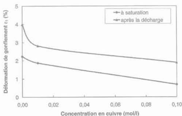
FIG. 4 Perméabilité en fonction de la concentration en cuivre dans la solution injectée et en fonction du système d'injection.
