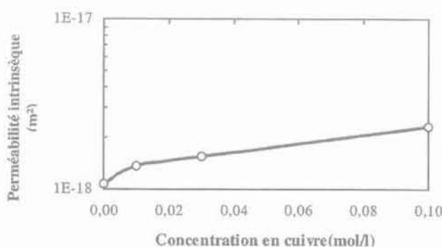
FIG. 9 Évolution de la perméabilité intrinsèque de la Fo-Ca en fonction de la concentration en cuivre. Evolution of the Fo-Ca intrinsic permeability versus copper concentration.
