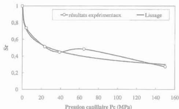
FIG. 8 Exploitation des paramètres mesurés pour la Fo-Ca en vue d'une modélisation du transfert de masse : a) exemple de lissage de courbe de rétention par une fonction hyperbolique pour la Fo-Ca infiltrée à l'eau ; b) évolution du coefficient de la loi en fonction de la concentration en cuivre. Evolution of the Fo-Ca parameters for mass transfer modelling : a) example of retention curve fitted by an hyperbolic function for Fo-Ca soaked with water ; b) evolution of coefficient of the S_r = f(P_c) curve versus copper concentration.
