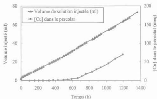
FIG. 2 Réponse de l'argile Fo-Ca à l'injection d'une solution à 10^{-1} mol/l de nitrate de cuivre en fonction du temps avec l'œdomètre à seringue : a) évolution du volume injecté et de la déformation de gonflement axiale ; b) évolution du volume injecté et de la concentration en cuivre dans le lixiviat. An example of solute intake with [Cu^{2+}] = 10^{-1} mol/l versus time using the syringe oedometer; a) evolution of solute intake and swelling axial strain; b) evolution of solute intake and copper concentration in leachate.
