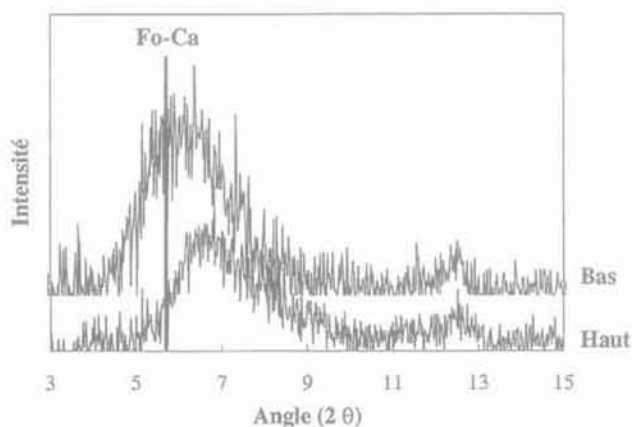
FIG. 3 Évolution des spectres de diffraction des rayons X de la Fo-Ca après 1 360 heures d'infiltration par une solution de nitrate de cuivre à 10^{-1} mol/l en fonction de la zone de prélèvement en comparaison avec le spectre de la Fo-Ca matérialisée par une droite d'abscisse 5,7 degré en 2\theta .
