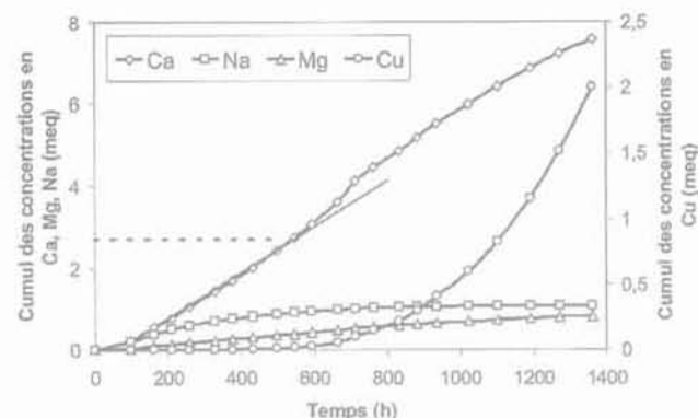
FIG. 7 Évolution du cumul des concentrations des ions \text{Ca}^{2+} et \text{Cu}^{2+} dans le percolat en fonction du temps.
