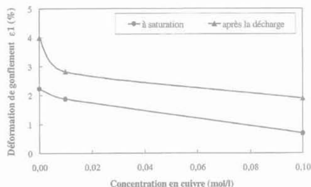
FIG. 6 Déformations de gonflement de l'argile en fonction de la concentration en cuivre dans la solution avec l'oedomètre à seringue ; comparaison entre la déformation obtenue à saturation et celle obtenue après la décharge hydromécanique en fin d'essai.
