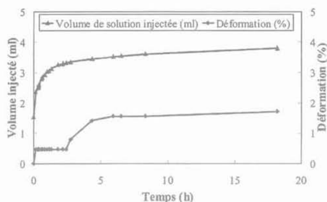
FIG. 2 Réponse de l'argile Fo-Ca à l'injection d'une solution à 10^{-1} mol/l de nitrate de cuivre en fonction du temps avec l'œdomètre à seringue : a) évolution du volume injecté et de la déformation de gonflement axiale ; b) évolution du volume injecté et de la concentration en cuivre dans le lixiviat. An example of solute intake with [Cu^{2+}] = 10^{-1} mol/l versus time using the syringe oedometer; a) evolution of solute intake and swelling axial strain; b) evolution of solute intake and copper concentration in leachate.
