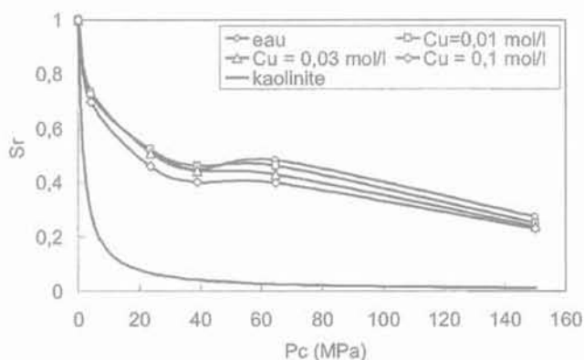
FIG. 5 Courbes de rétention après pollution de l'argile avec des solutions de nitrate de cuivre.
