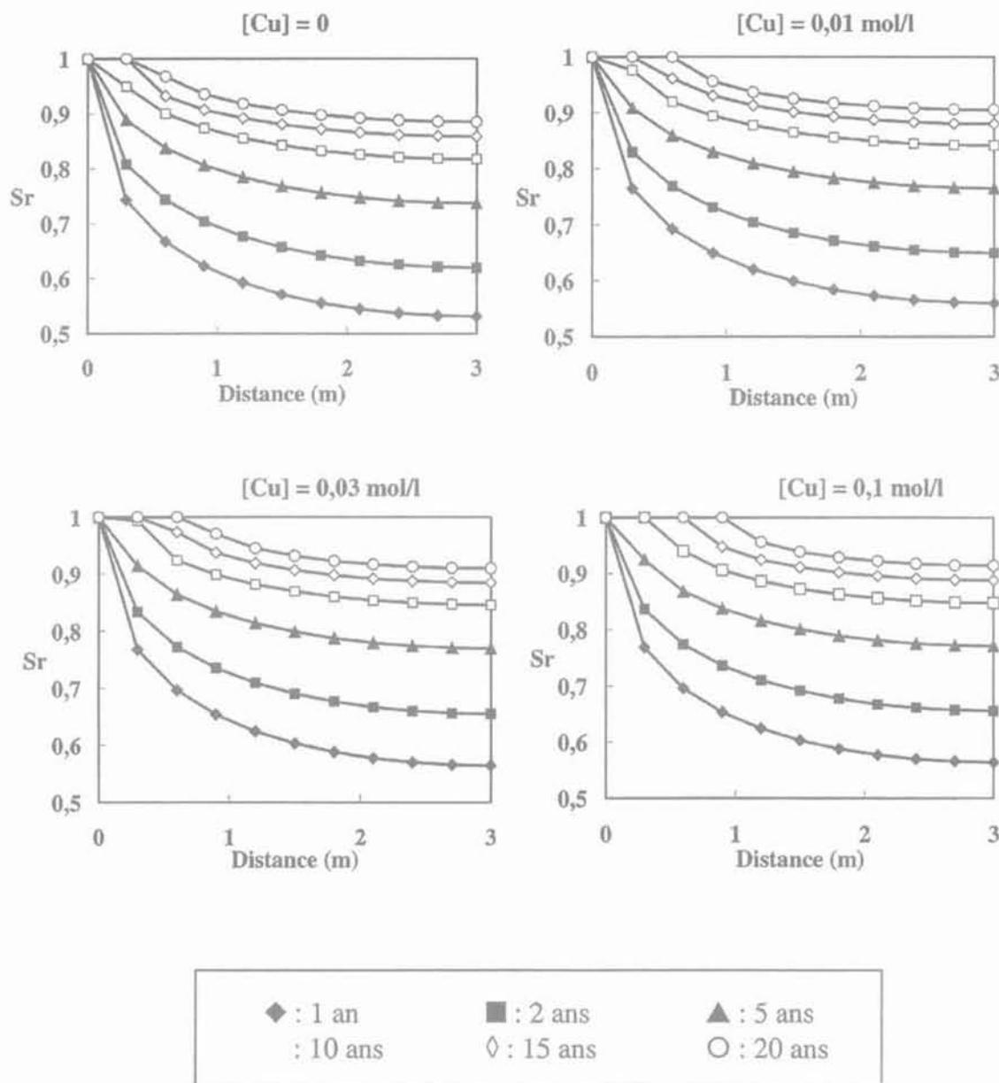
FIG. 10 Simulations de la cinétique de saturation en eau à l'échelle d'un massif d'argile de 3 m de longueur après pollution avec des solutions de nitrate de cuivre. Simulation of the water saturation kinetics through a 3 m long clay polluted (with copper nitrate solutions) medium.
