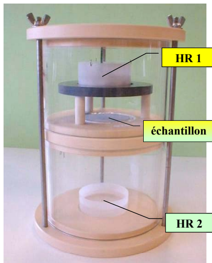
Figure 9 : cellule de diffusion
