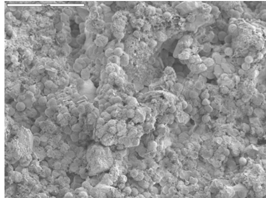
Figure 4 : Photographie MEB (échelle : 100 μm) montrant la diversité de porosités (Rautureau [3])
