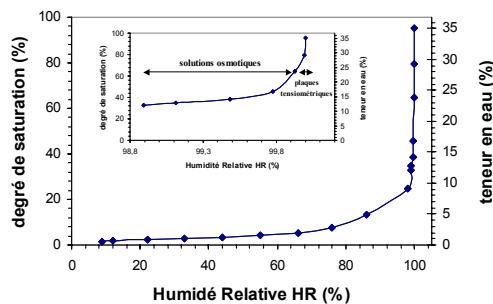
Figure 5 : Courbe de rétention d'eau suivant l'humidité relative
