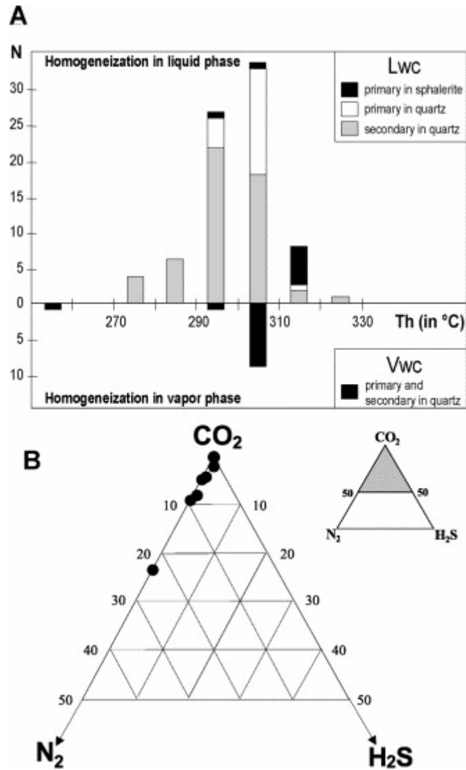
Fig. 3. (A) Distribution of the homogenization temperatures ( T_h in °C) of the different observed fluids. (B) Ternary CO 2 -H 2 S-N 2 diagram showing the composition of the gaseous phase for the Vw-c fluids. See text for details. (A) Distribution des températures d'homogénéisation des différents types de fluides rencontrés. (B) Diagramme ternaire CO 2 -H 2 S-N 2 montrant la composition de la phase gazeuse des inclusions fluides de type Vw-c. Voir texte pour les détails.
