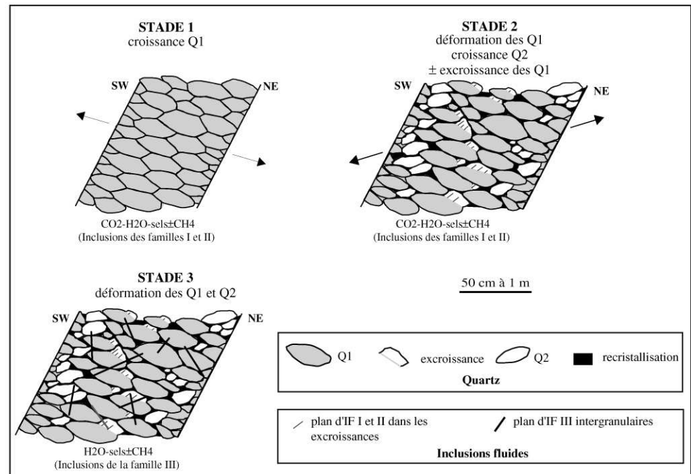
Figure 4. Modèle de formation des veines de quartz aurifère du district de Lo Inceivable.
