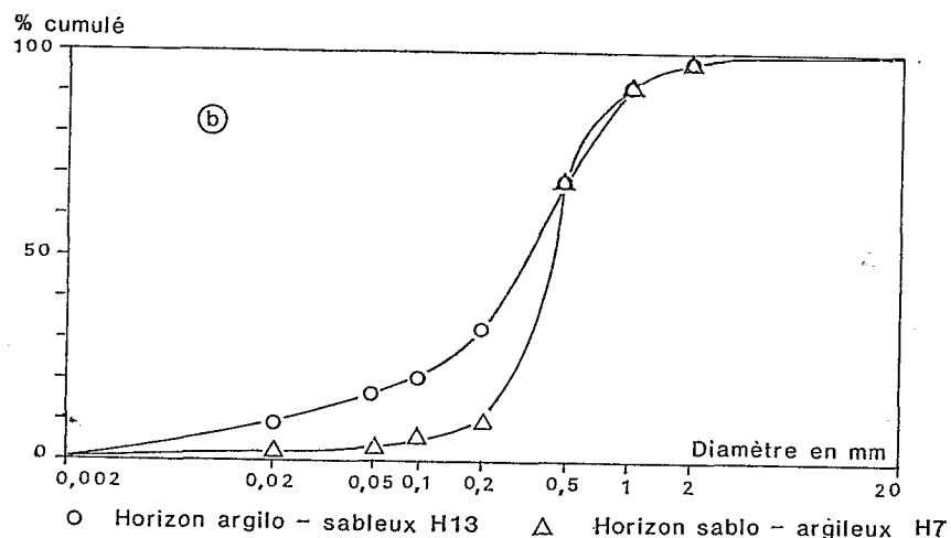
Figure 7 : Courbes granulométriques cumulatives des fractions 0,02-20 mm. Horizons appartenant à un profil de sol du domaine amont (a) et à un profil de sol du domaine sommital (b).
