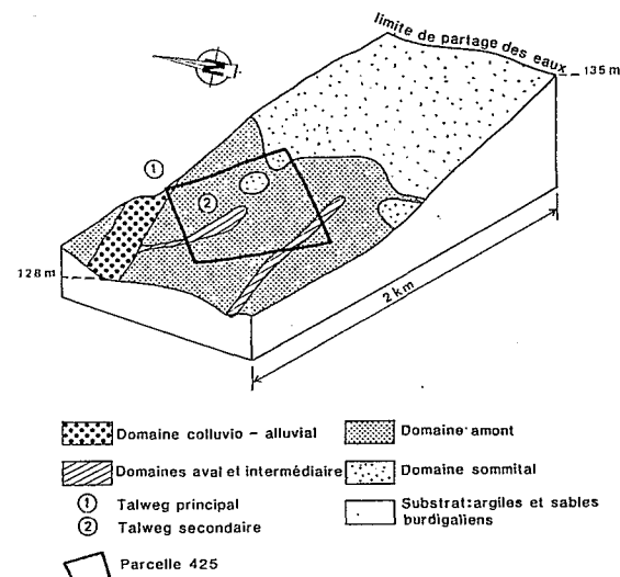
Figure 2 : Les différents domaines pédologiques sur le versant. The pedological fields on the slope.
