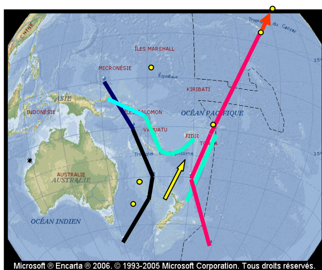
Fig. 11. Interférences aux antipodes en -214 Ma projetées sur une carte actuelle. Y figurent aussi les fosses existantes (en Cyan) et les points chauds (points jaunes) : Tasmanid, Lord Howe, Samoa, Hawaii, Caroline.
