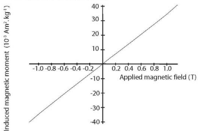
Boisset Pluton (49)
