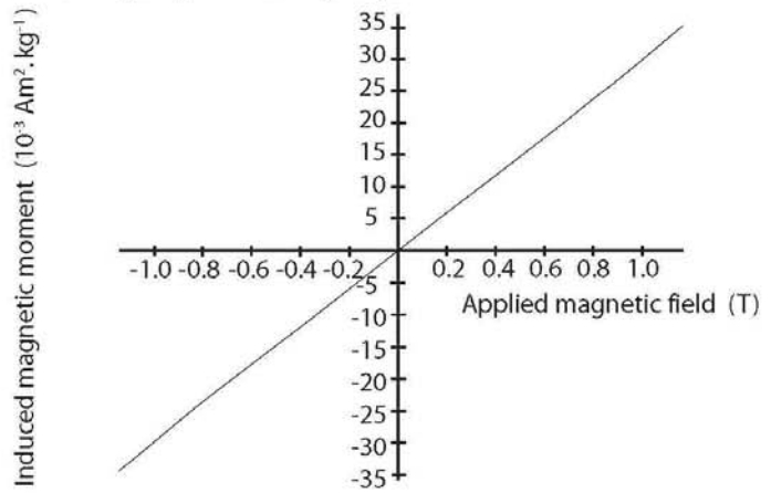
Omps pluton (32)
