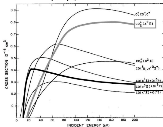
Figure 2 : Sections efficaces de dissodes molécules de CO_2 produisant les états excités de CO ( a^3\Pi ) (traits plein noir) et de CO_2^+ ( B^2\Sigma_u^+ ) (trait plein en gris). D'après [12].
