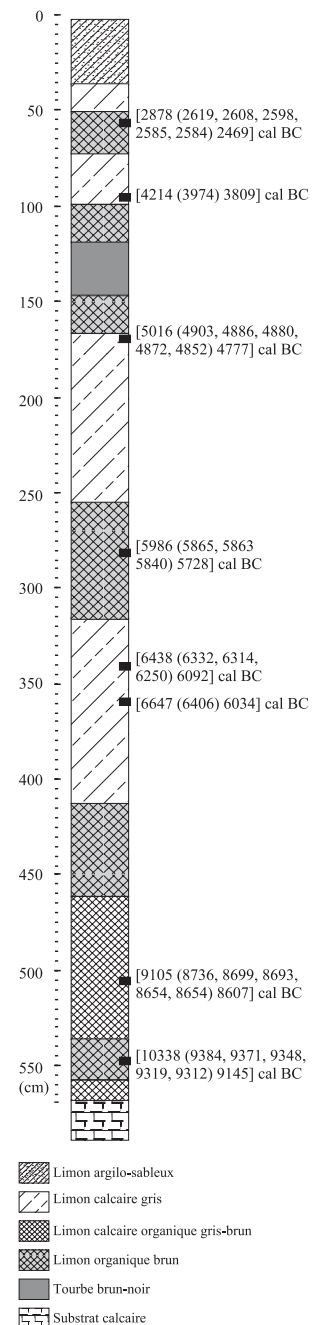
Figure 4 : Lithologie et datations radiocarbone du forage du "Marais du Grand-Chaumet" (Saint-Aoustrille, Indre, France).
