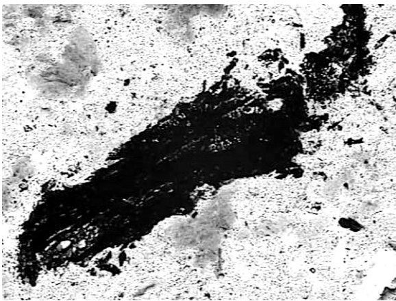
Figure 6 : Marais du Grand Chaumet (Saint-Aoustrille, Indre). Exemple d'observations microscopiques de micro-charbons de bois sur les lames minces en lumière transmise (1 et 2) et sur des lames polies en lumière réfléchie (3 et 4).
