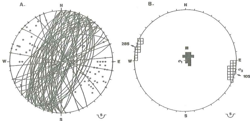
Figure 2A - Projection stéréographique des plans de failles synsédimentaires (Schmidt, hémisphère inférieur)
