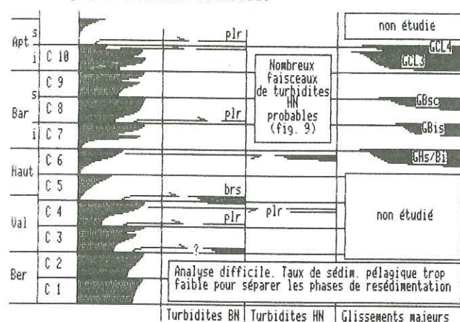
Fig. 8 : Calage biostratigraphique par les ammonites des cycles eustatiques du Crétacé inférieur, du Berriasien à l'Aptien inférieur. La biozonation utilisée est celle de la "Synthèse du Sud-Est" (R. Busnardo, in Debrand-Passard et al., 1984), légèrement modifiée à la limite Barrémien inf./sup. (1): renseignement oral de R. Enay. Un autre exemple de la coïncidence entre phénomènes sédimentaires et "renouvellements" des faunes d'ammonites est détaillé par ailleurs dans ce volume (Atrops et Ferry) et éclaire la manière dont les cycles ont été définis dans le Crétacé inf.
