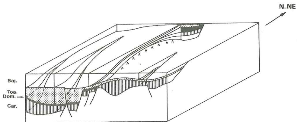
Fig. 5 - Déformations anté-bathoniennes dans Les Rochers de Hongrie Ante-Bathonian deformations in the Rochers de Hongrie
