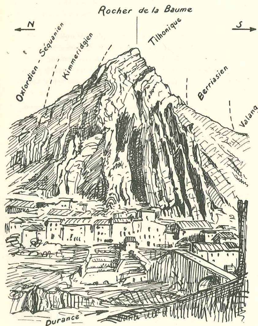
FIG. 6. — LA CLUSE DE SISTERON, DANS LES CALCAIRES TITHONIQUES. Dessin d'après une photogr. de W. KILIAN prise de la Citadelle.
