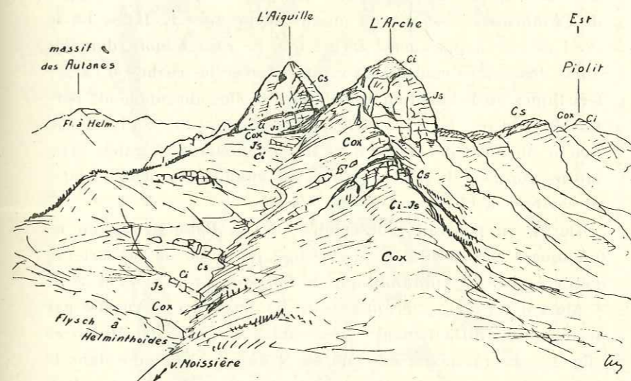
FIG. 13. — ÉCAILLES SUBBRIANÇONNAISES DU VERSANT W DU MASSIF DE PIOLIT, VUES DU COL DE MOISSIÈRE.
