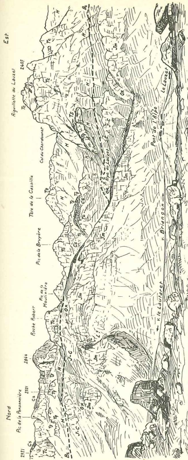
FIG. 27. — PANORAMA DES MONTAGNES DE LA RIVE GAUCHE DE LA GUISANE, AU LAUZET, ENTRE LE MONÉTIER-LES-BAINS ET LE LAUTARET, MONTRANT LE CHEVACHEMENT DE LA ZONE DU BRIANÇONNAIS SUR LA ZONE SUBBRIANÇONNAISE.
