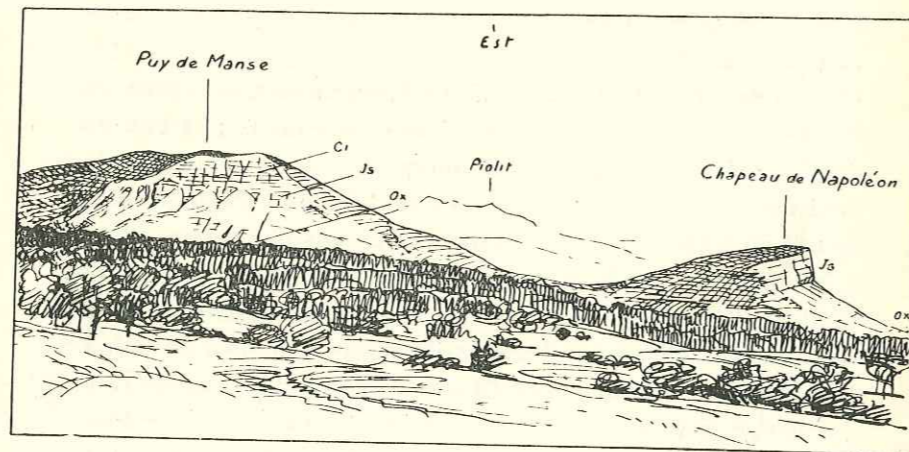
FIG. 11. — ECAILLES ULTRADAUPHINOISES DU PUY DE MANSE ET DU CHAPEAU DE NAPOLEON (OU SOMMET DE LA ROCHETTE). Vue prise de la route un peu au SW du Col de Manse. On remarquera l'extrême réduction d'épaisseur de la série Malm (Js) - Crétacé inf. (Ci) surmontant les terres noires (Ox).
