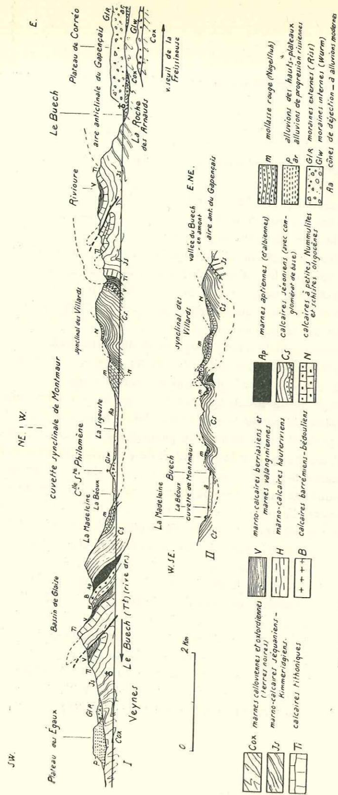
FIG. 10. — COUPES SCHEMATIQUES A TRAVERS L'EXTRÉMITÉ S DU DÉVOLUY, DANS LA CLUSE DE VEYNES. I. — Profil des montagnes de la rive droite. II. — Coupe de détail de la rive gauche (d'après P. LORY).
