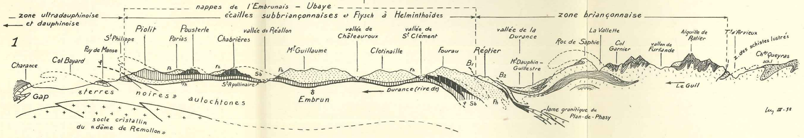
PL. VII. — Coupes géologiques schématiques montrant la structure d'ensemble des nappes de l'Embrunais et du Briançonnais. FIG. 1. — Profil W-E des montagnes de la rive droite de la Durance entre Gap et Montdauphin et de la rive droite du Guil entre Montdauphin et Château-Queyras. FIG. 2. — Profil NE-SW parallèle à la Durance dans les montagnes de la rive gauche vers le front des nappes de l'Embrunais. FIG. 3. — Coupe transversale de la région frontale des nappes briançonnaises au droit de la Tête de Gaulent. FIG. 4. — Coupe un peu plus au N, passant en aval de l'Argentière, et montrant la fenêtre de l'Argentière et la digitation supérieure de Pierre-Eyraudz (Pic du Bonhomme). FIG. 5. — Coupe encore un peu plus au N, passant près du confluent Gyronda-Durance, et montrant le renversement de l'anticlinal de nappes de la fenêtre de l'Argentière, dans laquelle apparaît la zone subbriançonnaise.
