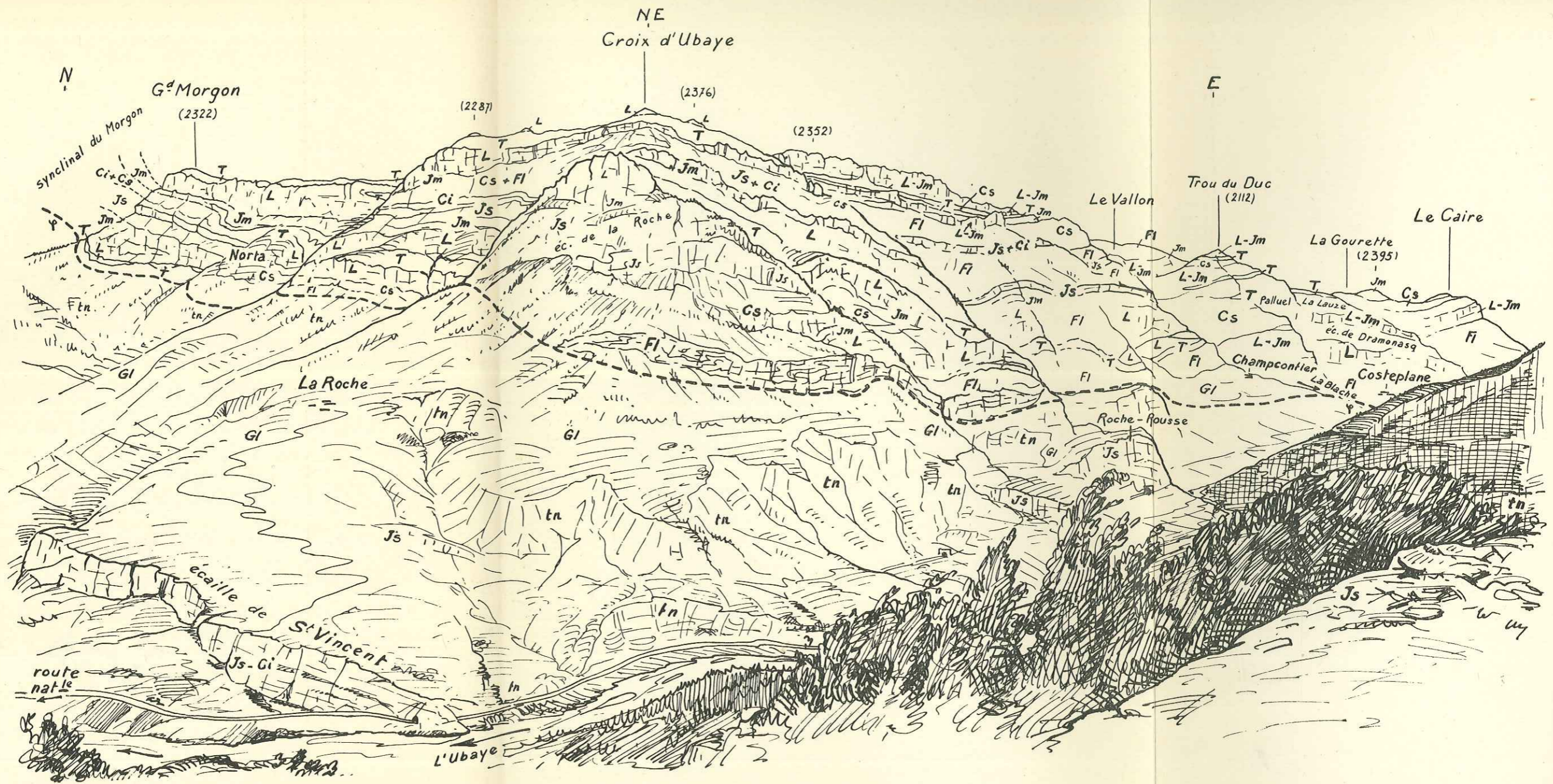
PL. VI. — LA FACE SW DU MASSIF DU MORGON, VUE DU TUNNEL DE SAINT-VINCENT, ROUTE BARCELONNETTE-DIGNE. Indications géologiques d'après D. SCHNEEGANS.
