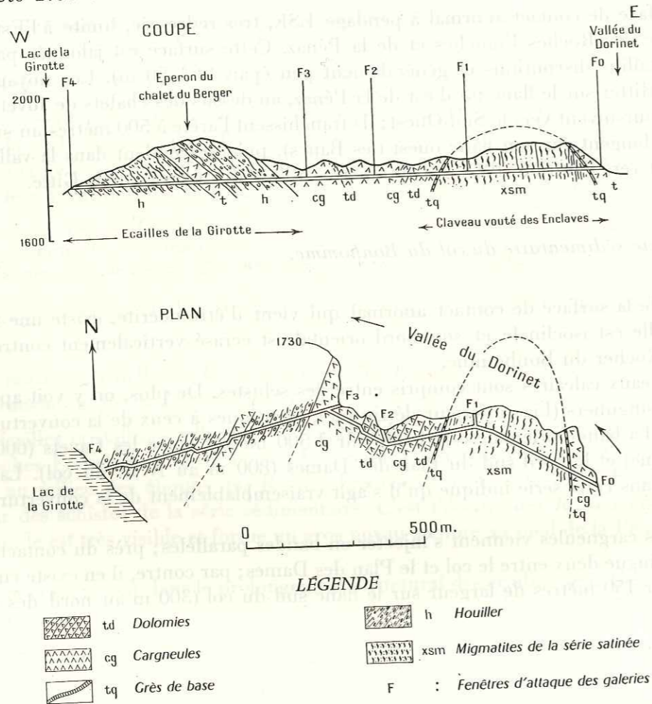
FIG. 24. — Coupe et plan géologiques de la galerie de Colombe.
