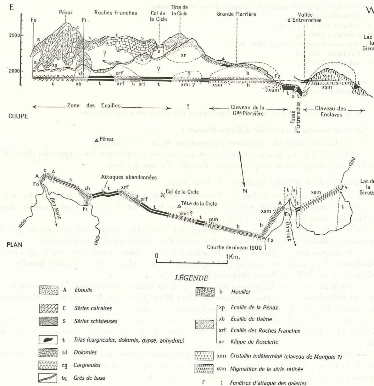
FIG. 25. — Coupe et plan géologiques de la galerie Bon Nant-Girotte.
