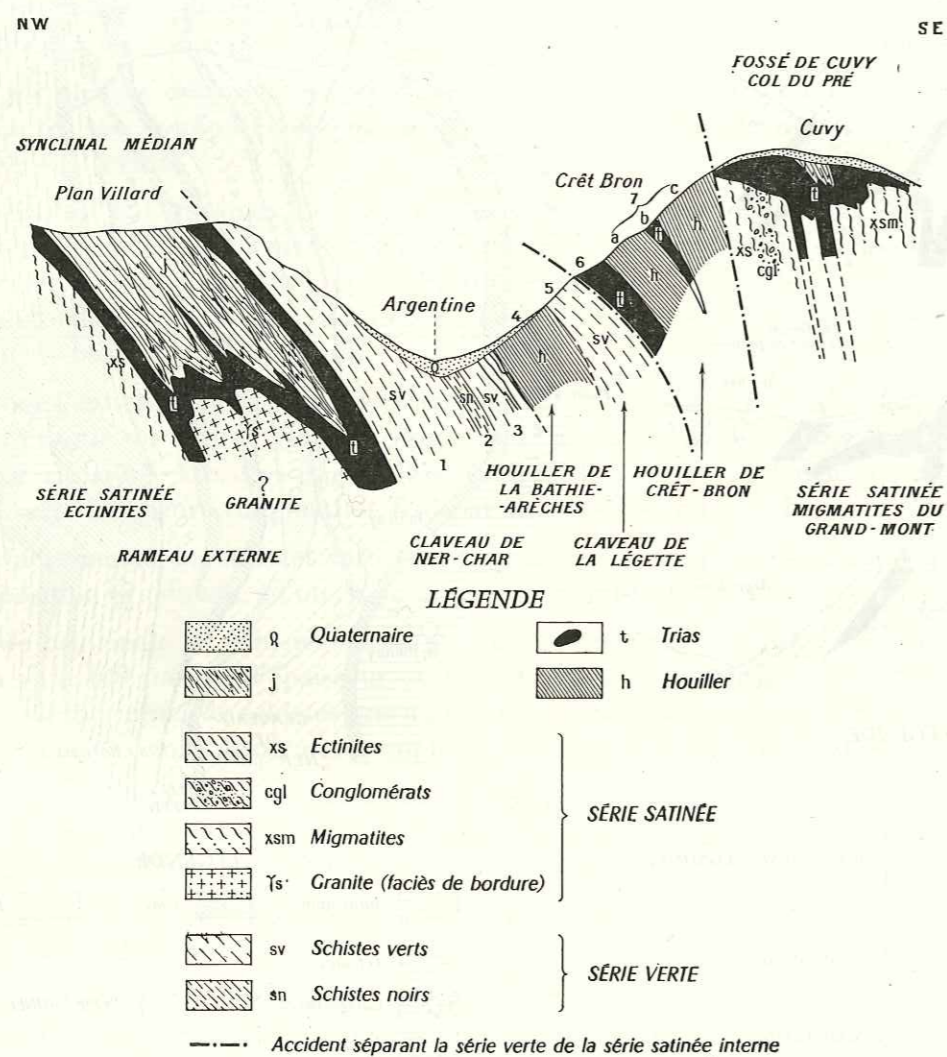
FIG. 28. — Coupe schématique à travers la zone des écaillles de Crêt Bron. (Interprétation.)
