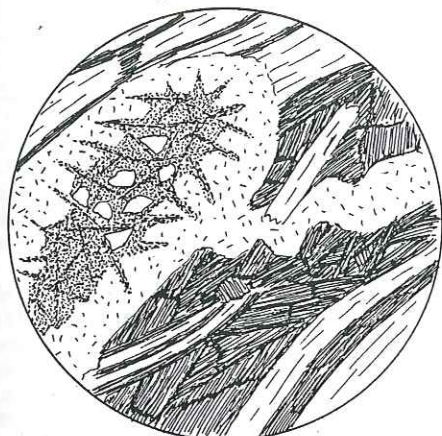
Fig. 34. Staurotide remplacée par de la séricite et des aiguilles de chloritoïde; au centre, des restes de staurotide (en blanc). Biotite et mica blanc. Arête W de la Croix de Tsousse.
