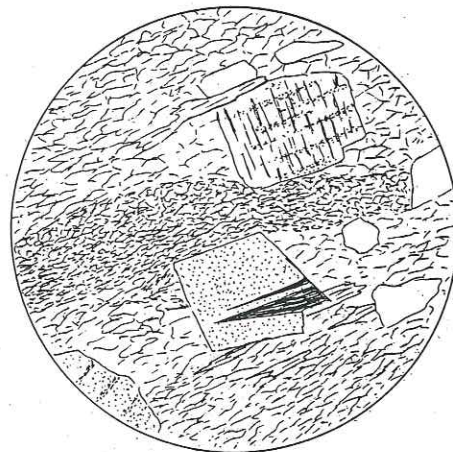
Fig. 86. Albites presque idiomorphes dont une avec maclé en échiquier, dans quartz, albite, mica blanc. Tuf volcanique du Grand Laget.
