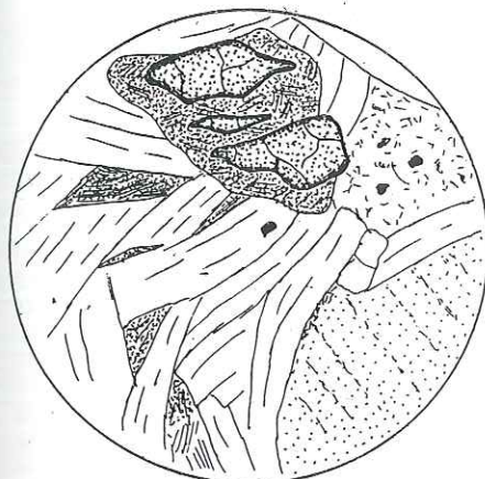
Fig. 24. Micaschiste avec grenat fortement altéré en chlorite, accompagné par de l'albite, de la séricite, du mica blanc et de la chlorite. La Tsarrette, pt.2190,5.
