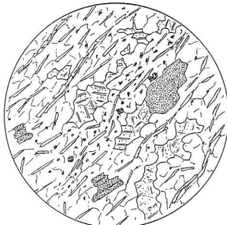
Fig. 64. Galet de quartzite calcifère des conglomérats. Quartz, mica blanc, chlorite, calcite, opaques. Goli des Otanes.
