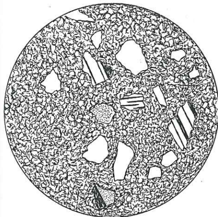
Fig. 66. Tuf volcanique vu en lumière polarisée. Matrice submicroscopique, grandes albites, quartz et mica blanc. Paroi E de la Chaudière
