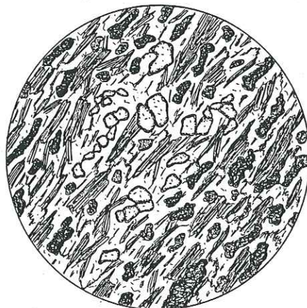
Fig. 49. Amphibolite rétro-morphosée. Fond d'albite, cristaux de chlorite et d'épidote accompagnés de fragments de grenats. Les Tsenas, rive droite du Valsorey.
