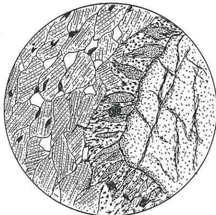
Fig. 127. Amphiboles bleues, radiaires sur un grenat; albite, épidote et grandes amphiboles vertes. Fournoutse
