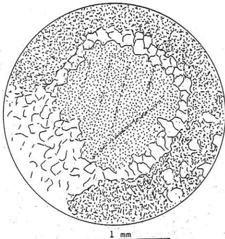
Fig. 135. Albite au coeur altéré et aurolé de petites albites (perpendiculaire à L) Mont Brûlé.
