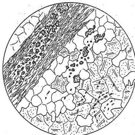
Fig. 53. Roche verte finement rubanée. Lit foncé d'actinote, chlorite et épidote. Lit clair de calcite, albite et épidote. Pte. des Trois Lacs, pt. 2580.
