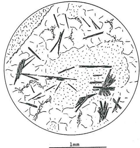
Fig. 124. Paillettes de stilpnomélane recoupant toutes les structures. Mont Brûlé.
