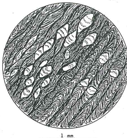
Fig. 88. Albites emprisonnant une ancienne schistosité, mica blanc et graphite. Z. Houillère, Chaux des Planards, pt. 2578.
