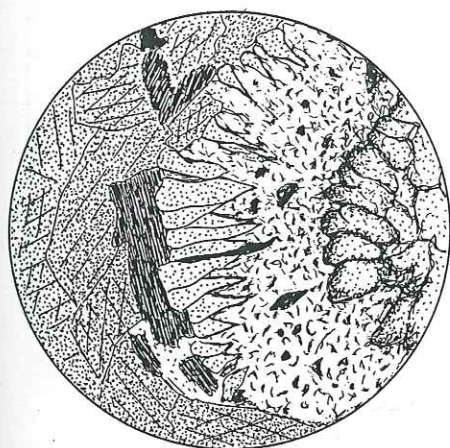
Fig. 9. Bordure d'altération d'un grenat, avec amphiboles bleues radiaires dans une matrice de chlorite, albite, épidote et m. op. de l'alpage de Fournoutse.
