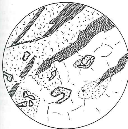
Fig. 18. Micaschite. Dans une matrice de quartz et de séricite grossière, grandes biotites et grenats en atoll. Torrent d'Allèves.
