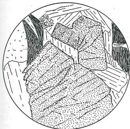
Fig. 26. Grands cristaux idiomorphes de staurotide accompagnés de biotite, de mica blanc et d'albite. Combe de Barasson.
