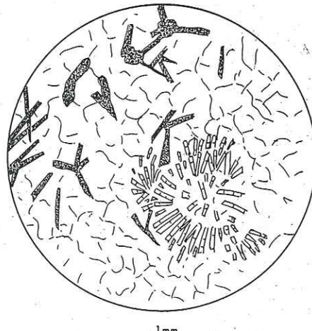
Fig. 132. Actinote et stilpnomélanes, fond de quartz. Mont Brûlé
