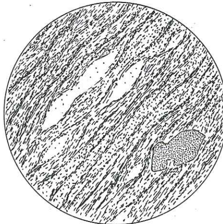
Fig. 81. Linéation minérale avec albites étirées. Mt. Brûlé.
