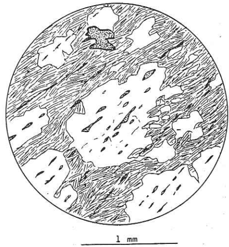
Fig. 112. Ovardite par rétrogenèse. Albite, chlorite. Crête de Menouve.
