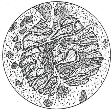
Fig. 8. Grenat altéré, mais ayant conservé sa forme. Dans le cristal, amphibole bleue et mica blanc. A la périphérie, actinote et séricite. E. de l'alpage de Fournoutse.
