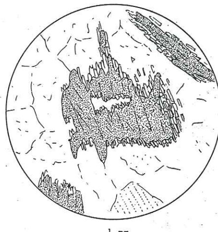
Fig. 130. Aiguilles d'actinote à la périphérie d'un glaucophane. Sommet de la Grande Chenalette.
