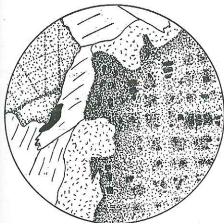
Fig. 28. Agrégat de minuscules cristaux d'altération préservant une ancienne structure. En haut à gauche une staurotide intacte. Mica blanc et séricite. Bourg St. Bernard.
