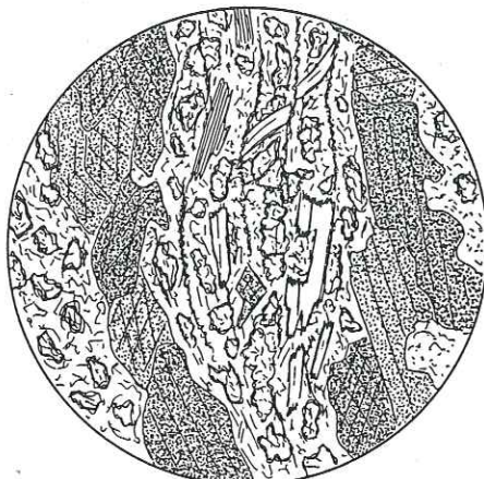
Fig. 126. Suite du processus et, par déformation, naissance d'un rubanement fin. Fournoutse.
