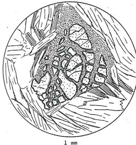
Fig. 98. Grenat altéré et chlorite. Fond de quartz, biotite et mica blanc. Une génération moule le grenat, l'autre le recourent. Plan de Tcholeire.
