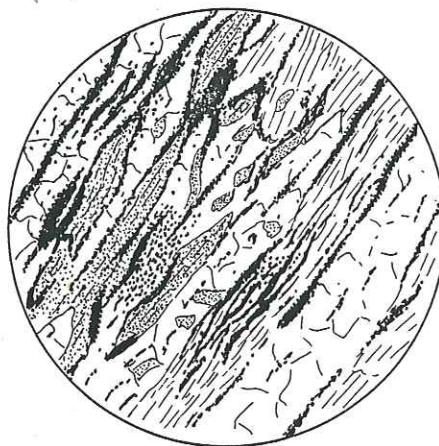
Fig. 15. Niveau graphiteux: quartz, albite, mica blanc, chlorite et graphite. Route de la Niord.
