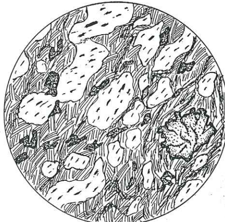
Fig. 128. Ovardite: albite, chlorite, mica blanc, épidote, sphène et gros grenat assez frais. Z. de Siviez, Challand d'en Haut.
