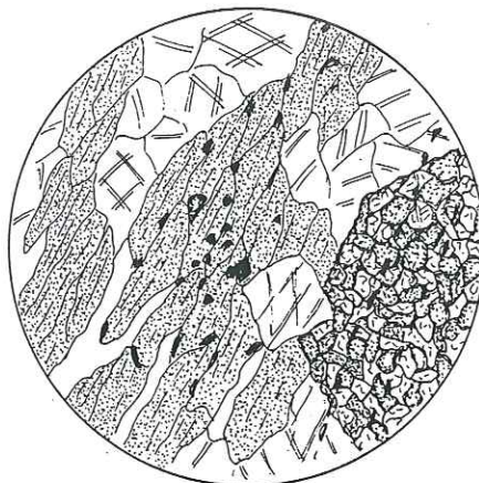
Fig. 35. Roche amphibolitique. Grands cristaux de hornblende, calcite, grenat altéré avec apparition de calcite et phyllosilicates. Minéraux opaques. Arête W de la Croix de Tsousse.
