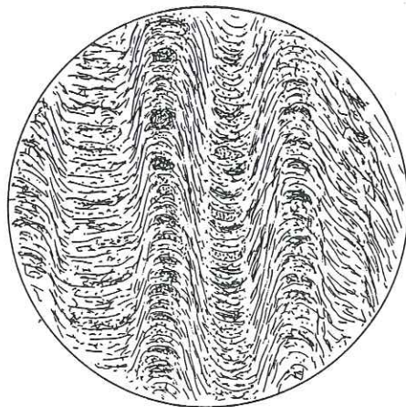
Fig. 80. Clivage de crénulation des plis récents. Goli des Otanes.
