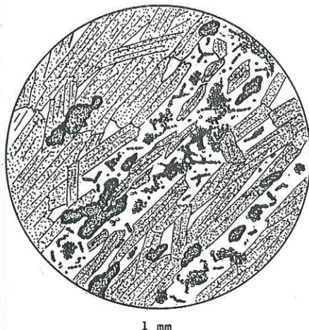
Fig. 30. Amphibolite très riche en hornblende, avec sphène, épidote en grains minuscules et albite limpide. Torrent de Perche.
