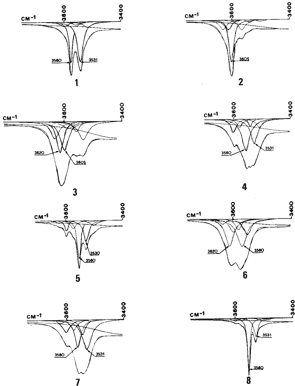
Figures IV A 1-8 : Décomposition des spectres I.R. (1) Céladonite 69 G ; (2) Leucophyllite 31 ; (3) Glauconite B. Patom ; (4) Glauconite 655 ; (5) Glauconite Taiheisan ; (6) Glauconite E 8/2 (7) Glauconite 5/1 ; (8) Céladonite Zavalye
