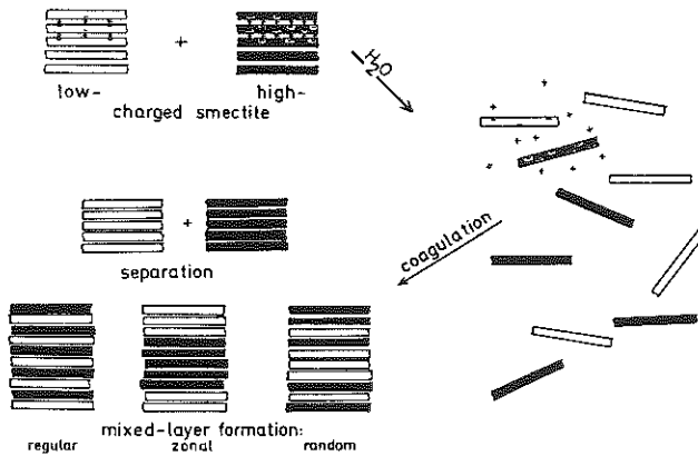
Fig.VI.3.2 Désagrégation de la montmorillonite sodique dans l'eau, formation d'une suspension colloïdale et réagrégation pour donner des cristaux (d'après Frey et Lagaly (1979 b))
