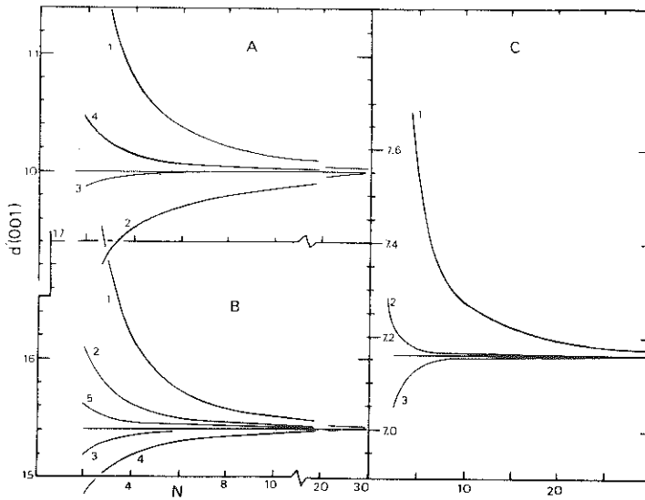
Fig.VI.3.1-Distances apparentes d(001) en Å déterminée à partir des diffractions 0001 l = 1-5 par cristal avec N feuillets A biotite B montmorillonite C kaolinite d'après Brindley (1980)
