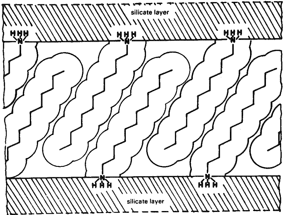
Fig .I2 : Structure de type paraffinique formée par les chaînes alkyl-ammonium dans l'espace interfoliaire des feuillets (d'après Lagaly et Weiss, 1969)
