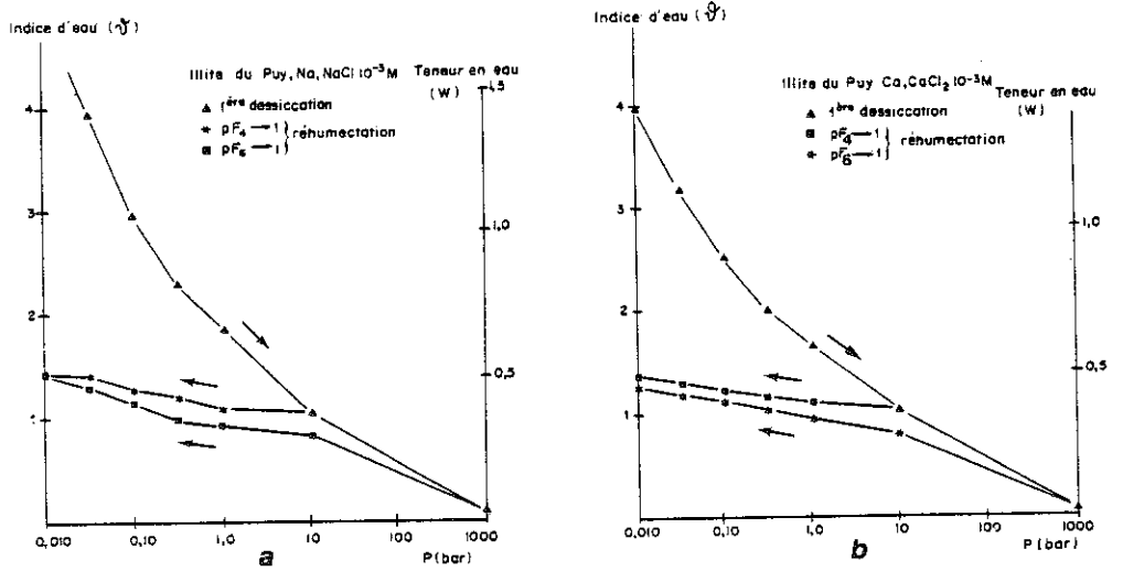
Fig.15 - Evolution de la teneur en eau de l'illite du Puy (a) Na, (b) Ca
