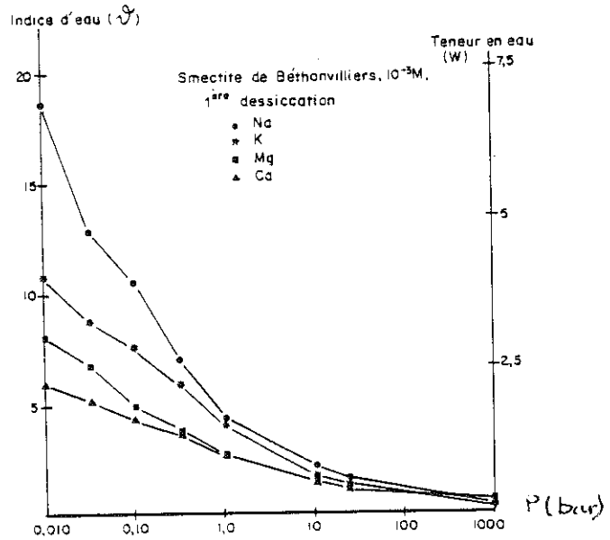
Fig. 9 - Evolution de la teneur en eau de la smectite de Béthonvilliers Na, K, Mg et Ca, 10^{-3} M au cours de la première dessiccation
