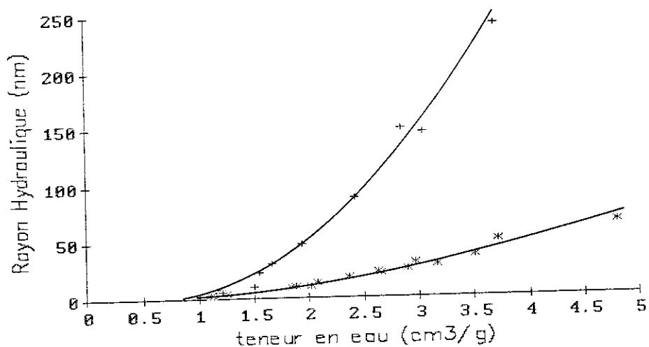
Fig. 18 - Courbes représentant le rayon hydraulique moyen en fonction de la teneur en eau dans le cas où l'hectorite-Ca est dispersée dans une solution 10^{-3} M en \text{CaCl}_2 (*) et 10^{-1} M en \text{CaCl}_2 (+).
