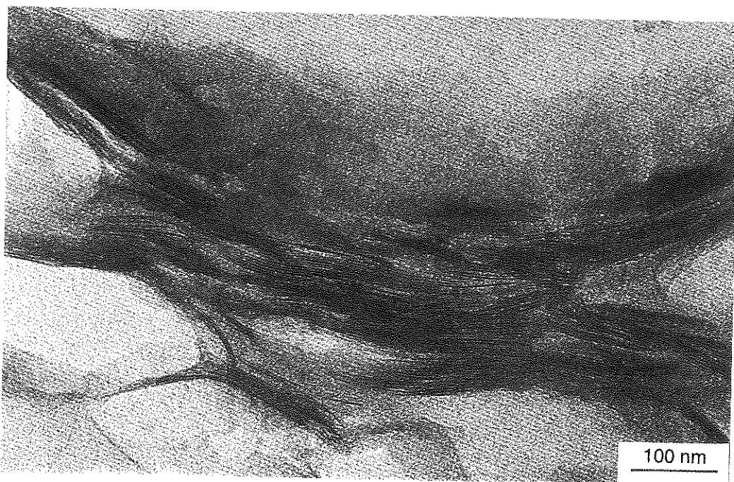
Fig.26 - Particule caractéristique d'une montmorillonite Ca (photo A.M. JAUNET)
