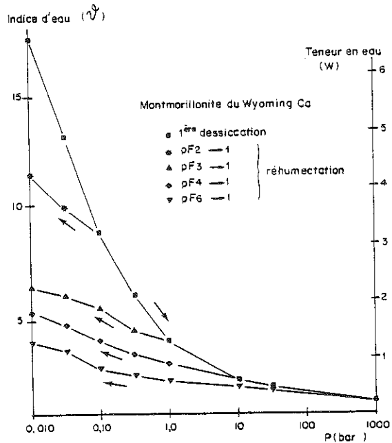
Fig. 14 - Evolution de la teneur en eau au cours de la dessiccation et de la réhumectation de la montmorillonite du Wyoming Ca, CaCl 2 10^{-3}M ; (■) 1 ère dessiccation ; (*) réhumectation de pF 2 à pF 1 ; (▲) pF 3 à pF 1 ; (◆) pF 4 à pF 1 et de (▼) pF 6 à pF 1
