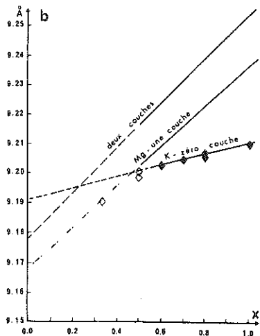
Fig. IV-1: Variation du paramètre b en fonction de la charge dans les saponites-K: ◆ valeur déterminée en fonction de la réflexion 060, 331; ◇ valeur déterminée à partir de la bande 06,33.
