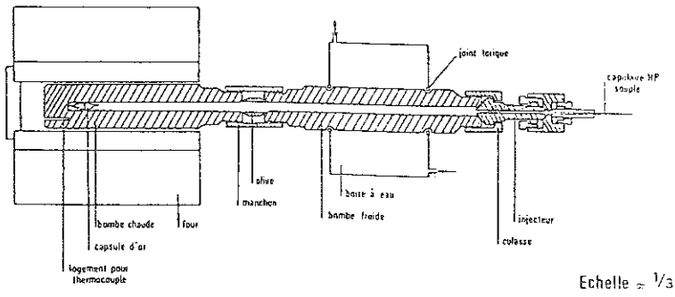
Fig.V-9 Autoclave pour synthèse à nucléation isotherme (Rudert et al., 1976)
