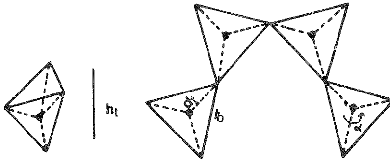
(a) Tétrahèdre et couche tétraédrique
