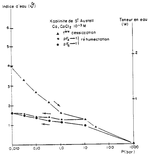
Fig.16 - Evolution de la teneur en eau de la kaolinite de St-Austell Ca ; (▲) 1 ère dessiccation (*) réhumectation de pF 4 à pF 1 (●) de pF 6 à pF 1
