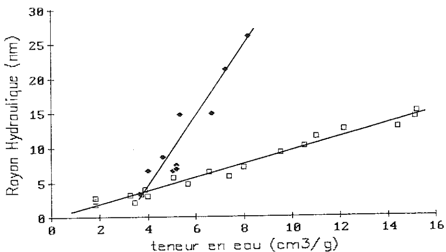
Fig. 19 - Courbes représentant le rayon hydraulique moyen en fonction de la teneur en eau dans le cas de la montmorillonite-Na dispersée dans une solution 10^{-3} M en \text{NaCl} (□) et 10^{-1} M en \text{NaCl} (♦).
