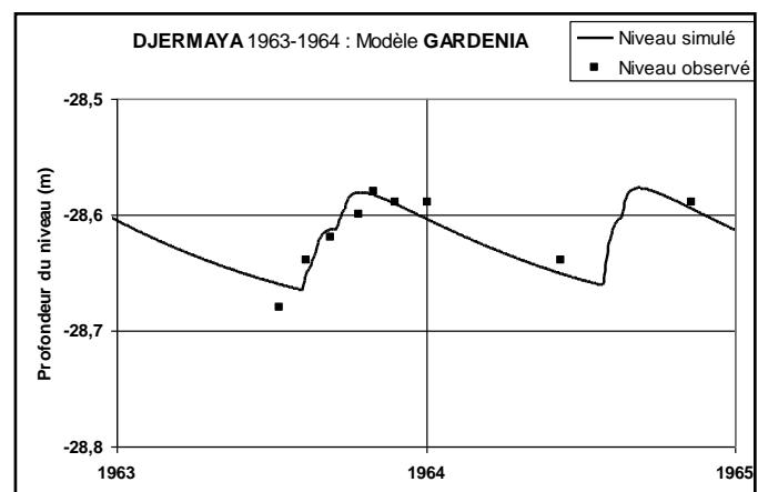
Fig. 3 – Djermaya. Modélisation des niveaux piézométriques 1963-1964. Fig. 3 – Djermaya. Modelling of the piezometric levels 1963-1964.
