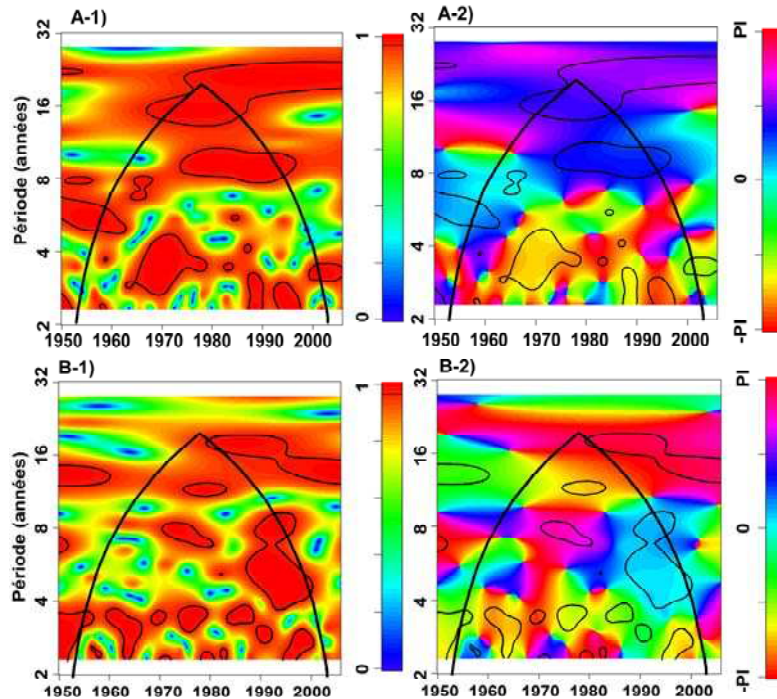
Figure 10.A.1(B.1) : spectre de cohérence par ondelettes entre l'indice TNA (TSA) et la pluviométrie à Maïné-Soroa sur la période 1950-2005. A.2(B.2) : spectre de phase associé (trait gras : cône d'influence ; traits fins : limite de confiance 90%).
