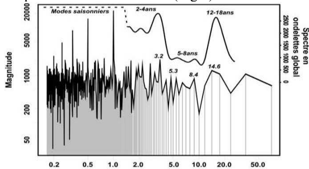
Figure 4 : Transformée de Fourier (données mensuelles) et spectre en ondelettes global des cumuls mensuels de précipitations à Mainé-Soroa sur la période 1950-2005.
