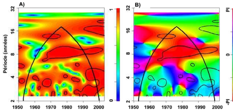
Figure 8.A(B) : spectre de cohérence (phase) par ondelettes entre la pression atmosphérique aux Açores et la pluviométrie à Maïné-Soroa sur la période 1950-2005. (trait gras : cône d'influence ; traits fins : limite de confiance 90%).
