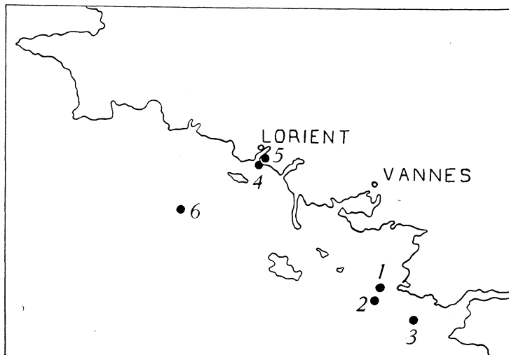
FIG. 1. — Gisements de Nummulites des côtes méridionales de Bretagne. — 1, plateau du Four ; 2, banc de Guérande ; 3, rochers de la Banche ; 4, pointe de Gâvre ; 5, tranchee de Locmalo ; 6, station 441, dragage du Président Théodore-Tissier .
