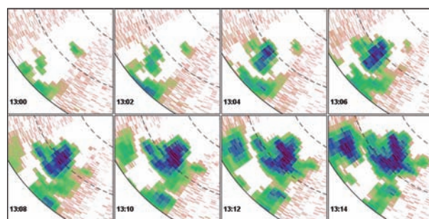
Figure 12 - Observations du radar en bande X situées sur le Bischenberg. Détail de l'évolution temporelle d'une cellule orageuse pour la journée du 12 août 2007 entre 13 h 00 TU et 13 h 14 TU.
