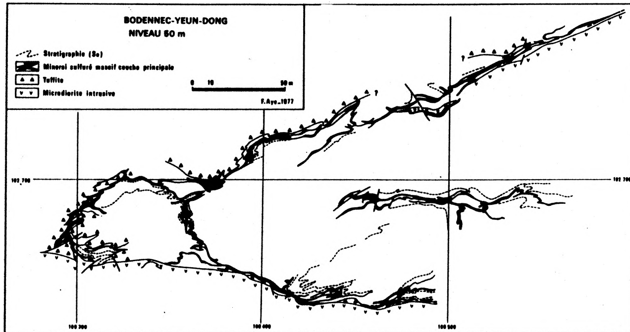
FIG. 4 - BODENEC-YEUN DONG - PLAN DU NIVEAU -50 M
