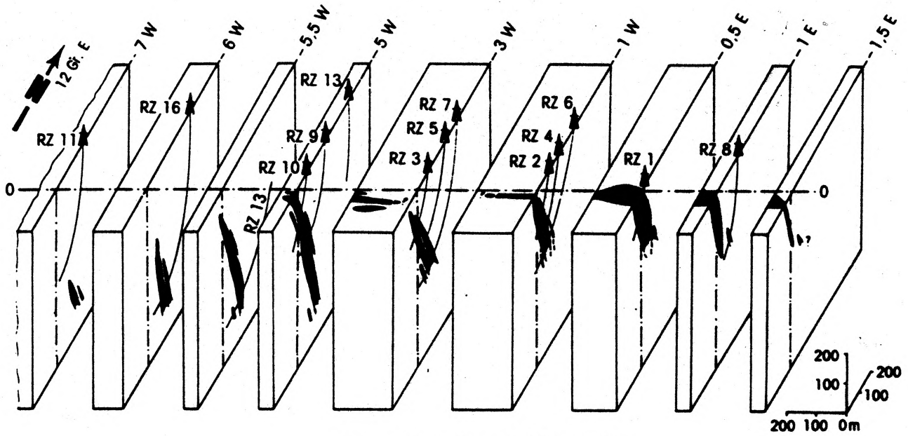
Coupes verticales éclatées, profils 7 Ouest à 1,5 Est.
