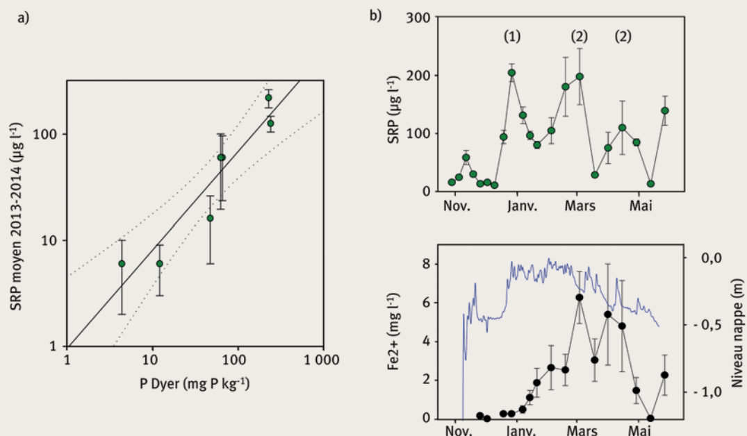
2 Relation entre teneur en P Dyer des sols et concentration moyenne en P dissous (SRP) dans l'eau du sol (a) et dynamique des concentrations en SRP et \text{Fe}^{2+} pour un piège à eau sélectionné à 15 cm de profondeur (b).
