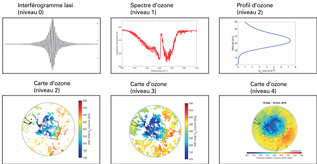
Figure 3. Les différentes étapes pour le traitement des données, du niveau 0 au niveau 4. L'exemple donné ici provient de la mission Iasi où la donnée initiale est un interférogramme (niveau 0) converti en spectre atmosphérique avec une transformée de Fourier (niveau 1), puis en profil vertical d'ozone à la localisation de la mesure (niveau 2). La carte globale d'ozone peut être présentée à la résolution des observations (niveau 2) ou sous forme de moyenne (niveau 3), avant d'être assimilée dans un modèle de chimie-transport (niveau 4).
