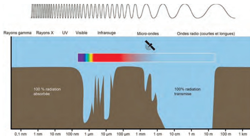
Figure 1. Gamme de longueurs d'onde couverte par le spectre électromagnétique, qui s'étend des rayons gamma aux ondes radios. Les ondes les plus et les moins énergétiques sont entièrement stoppées avant d'atteindre la surface terrestre. Le sondage de l'atmosphère par satellite repose sur les régions spectrales UV, visible, infrarouge, micro-ondes et radio. En particulier, les fenêtres atmosphériques optique et ondes radio sont exploitées pour sonder les couches les plus basses de l'atmosphère et la surface terrestre.
