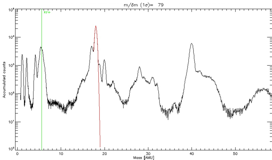
Fig. 56 Strofió mass range for two turns
