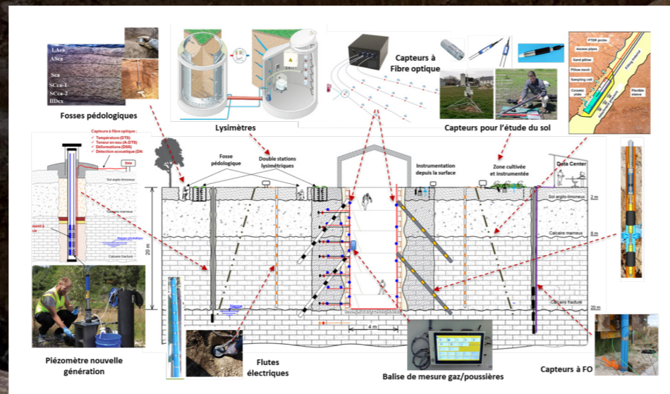
Schéma d'instrumentation scientifique du site O-ZNS (en surface, à travers le puits central et dans les forages environnants).
