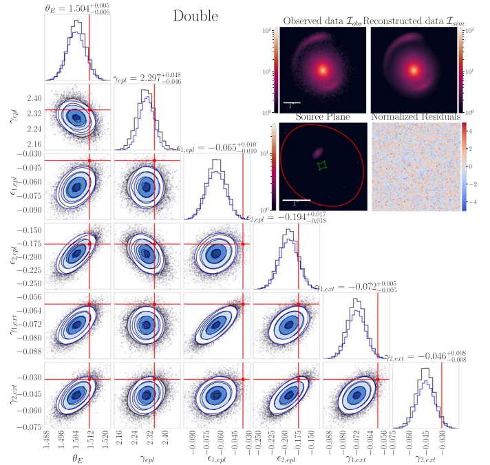
(d) Doubles
