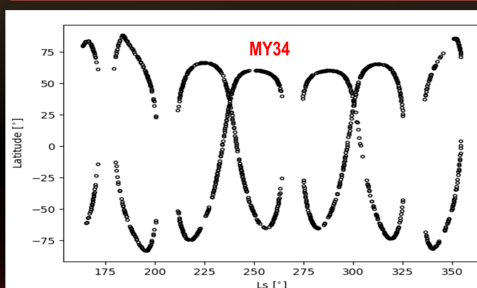
Fig.2 Latitude and Solar Longitude ( L_s ) data coverage for ACS-MIR.
