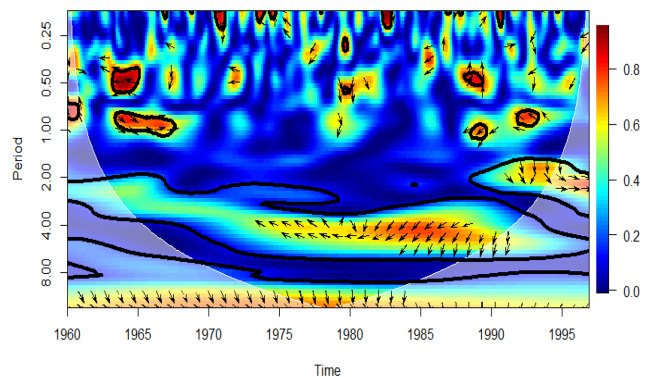
Figure 6. Cohérence en ondelettes entre l'indice ENSO et le débit à Tortiya amont.
