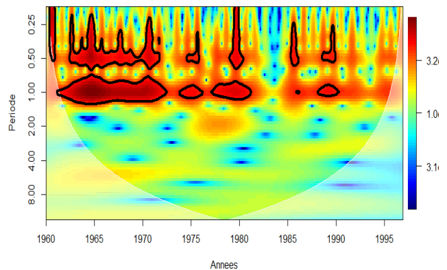
Figure 3. Analyse en ondelettes continues du débit à la station de Tortiya.
