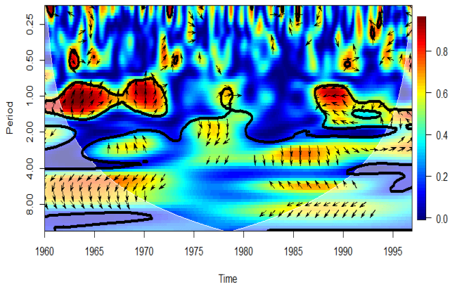
Figure 7. Cohérence en ondelettes entre l'indice NAO et le débit à Tortiya.
