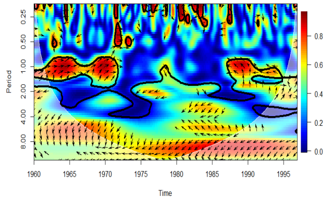
Figure 5. Cohérence en ondelettes entre l'indice NAO et la pluviométrie à Tortiya.
