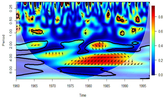
Figure 4. Cohérence en ondelettes entre l'indice ENSO et la pluviométrie à Tortiya.
