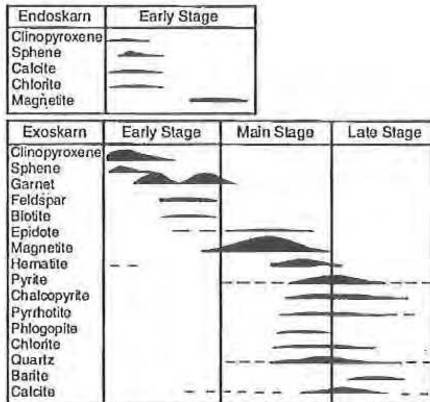
Figure 3.11 : séquence paragénétique des gisements des Beni Bou Ifrou, selon qu'il s'agisse d'endoskarn ou d'exoskarn (EL RHAZI & HAYASHI, 2002).
