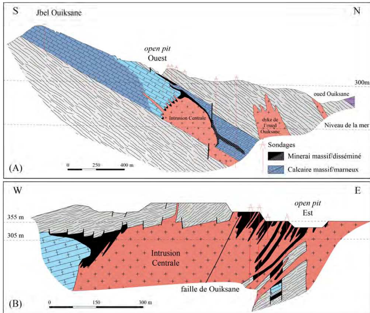
Figure 6.3 : coupes géologiques historiques explicitant la structure du gisement de Ouiksane (d'après RHODEN & ERENO, 1962). Le tracé de la coupe (A) est représenté sur la Figure 6.2 . La coupe (B) traverse d'Ouest en Est l' open pit .
