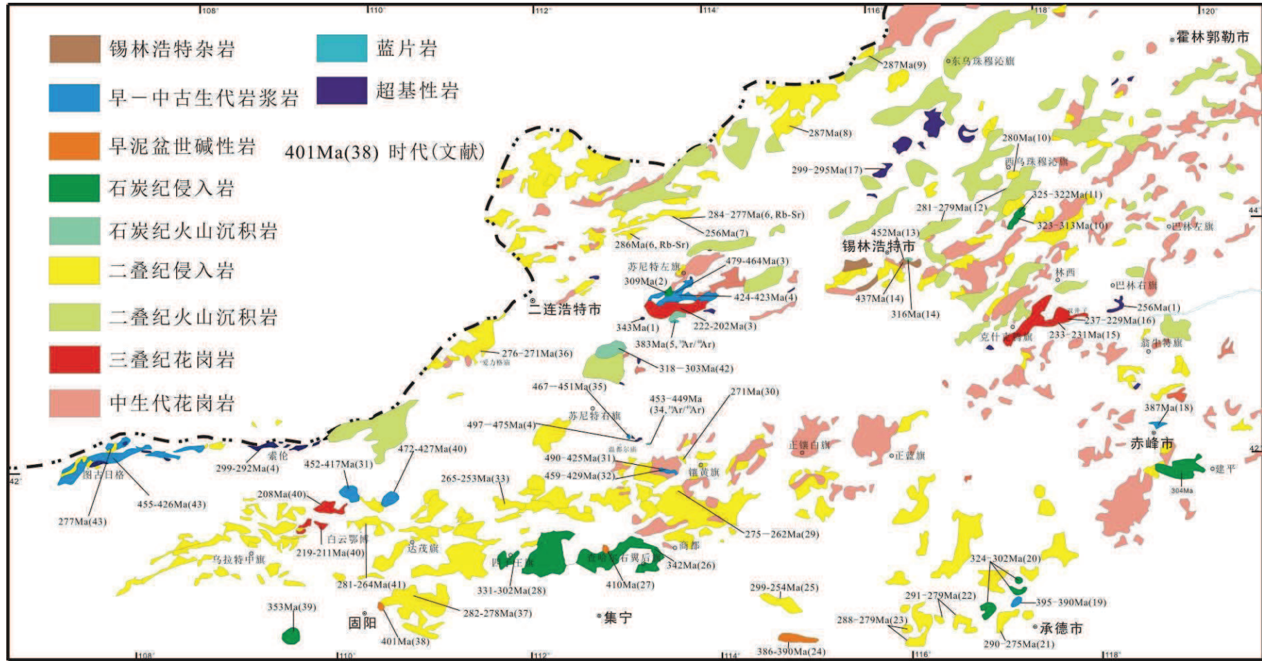
图2-3 内蒙古中部泥盆纪—二叠纪岩浆岩分布图
