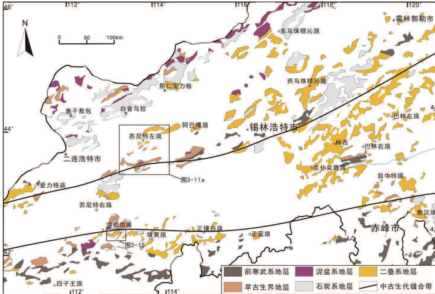
图2-2 内蒙古中东部古生代地层分布图 (内蒙古自治区地质矿产局, 1991)
