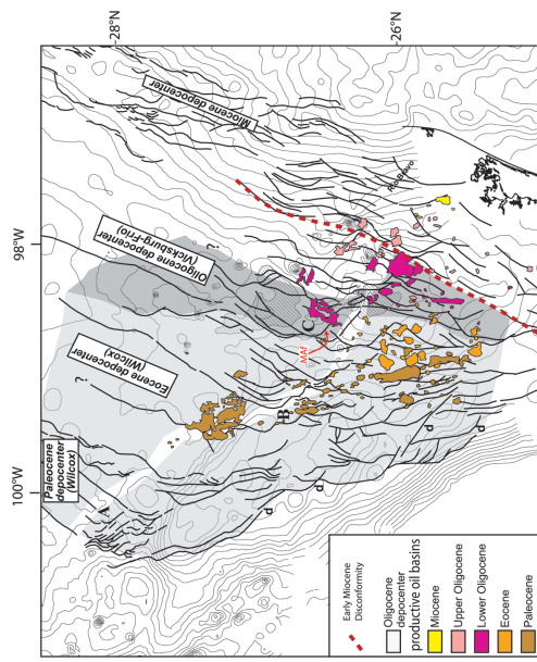
Fig. 6. — Surface trace for growth faults in the Burgos basin and localisation of the main oil spays classified by age (courtesy of PEMEX modified). Thin lines is gravimetric contouring of figure 7. MAF = Mac Allen fault area shown on fig. 9. A.B.C.D. see text for explanation. Note left lateral dragging of listric faults along the Rio Bravo fault. Dotted red line is the surface trace of the Early Miocene discontinuity, poorly affected by strike slip motion. cf. disconformity at the base of the Burgos basin. Fig. 6. — Tracé en surface des failles de croissance dans le bassin de Burgos, et localisation des réservoirs pétroliers classés par âge (courtoisie de PEMEX, figure modifiée). Le contourage en arrière plan est celui des données gravimétriques de la figure 7. MAf = faille de Mac Allen détaillée sur la figure 9. A.B.C.D sont explicités dans le texte. Remarque l'enlacement en feu sensuse du tracé des failles listriques le long de la faille du Rio Bravo. La ligne rouge pointillée correspond à la trace en surface de la discordance Miocène inférieure peu affectée par le mouvement décrochant. d : discordance à la base du bassin de Burgos.
