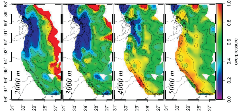
Fig. 8. – Overpressure state (0 is 100% hydrostatic and 1 is 100% lithostatic) at variable depths. Seawater density: 1030 kg m -3 ; sediment density: 2670 kg m -3 . Fig. 8. – Etat de surpression (0 correspond à 100 % hydrostatique et 1 à 100 % lithostatique) à différentes profondeurs. Densité de l'eau de mer : 1030 kg m -3 ; densité des sédiments : 2670 kg m -3 .
