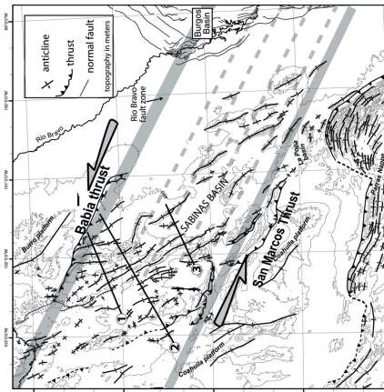
FIG. 11. – Structure sketch map of the left lateral shear band wrenching the Sabinas basin between the Rio Bravo fault and San Marcos fault. Topographic contours every 400 m. Dashed gray lines from figure 7, 1, 2, 3: location of sections figure 12. FIG. 11. – Carte structurale synthétique illustrant la bande de cisaillement sensière déformant le bassin de Sabinas entre les failles de Rio Bravo et de San Marcos. Contours topographiques tous les 400 m. Les lignes ponctillées grises proviennent de la figure 7, 1, 2, 3; localisation des coupes de la figure 12.
