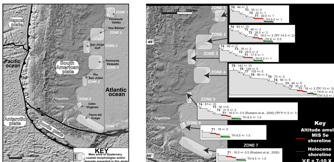
FIG. 3.1: Patagonie, zones principales d'échantillonnage (a) et profils topographiques moyens (b). Patagonia, main sampling zones (a) and elevation profiles (b).
