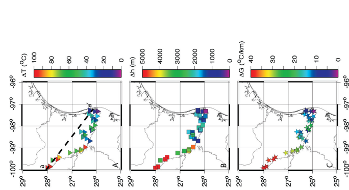
FIG. 3. – a) Difference between the current temperature and the maximum temperature recorded by the vitrinite in the sediments ( \Delta T , triangles); b) Equivalent maximum erosion \Delta h (squares); c) Equivalent maximum gradient change \Delta G (stars). Sampling depth ranges from 1500 m to 5000 m, aa': location of the cross-section, \Delta h is calculated assuming a constant gradient through time, identical to the present one; \Delta G is calculated assuming that the present burial depth is the maximum depth met by the sample. FIG. 3. – a) Différence entre températures actuelles et les températures maximales enregistrées par la vitrinite dans les sédiments ( \Delta T , triangles); b) Équivalent en érosion maximale \Delta h (carrés); c) Équivalent en changement de gradient \Delta G (étoiles). La profondeur d'échantillonnage varie de 1500 m to 5000 m, aa': localisation de la coupe sur la figure 4, \Delta h est calculé en supposant un gradient constant dans le temps; \Delta G est calculé en supposant que la profondeur d'enfouissement actuelle est la profondeur maximale connue par l'échantillon.
