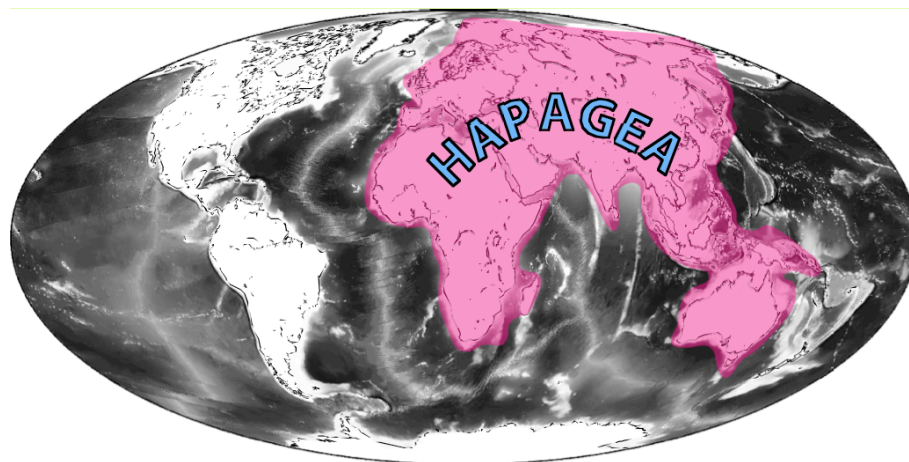
FIG. 4.1: Aggrégation actuelle des continents en un supercontinent : Hapagea. Present-day continental aggregation towards a supercontinent : Hapagea.
