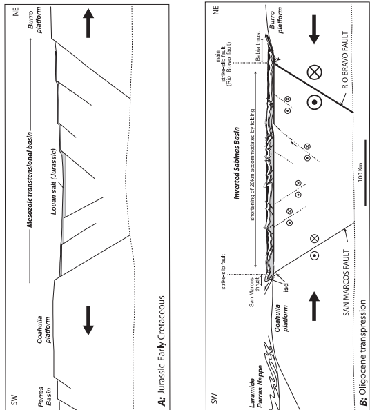
FIG. 13. – Schematic section of the Sabinas basin and its margins. A: before Oligocene inversion. B: transpositional inversion in the basin. FIG. 13. – Section schématique du bassin de Sabinas et de ses marges. A: avant l'inversion Oligocène. B: après l'inversion en transpression.
