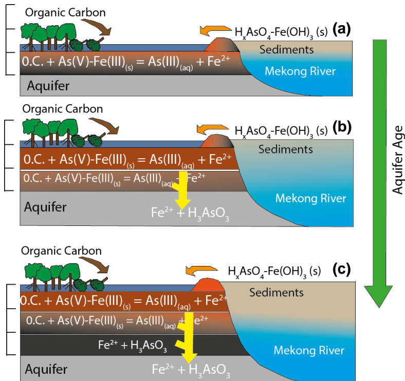
Figure Intr. 5 : (a) Lors des crues du Mékong, les oxydes de Fe porteurs d'As sont déposés dans les zones humides, l'apport de matière organique favorise la dissolution des oxydes de Fe, libère le Fe(II) et l'As(III). (b) Les apports du Mékong sont permanents et l'As(III) et le Fe(II) préalablement libérés migrent jusque dans les aquifères sous-jacents. (c) Continuité des phénomènes précédents avec les apports continus provenant du Mékong (Kocar, 2008)
