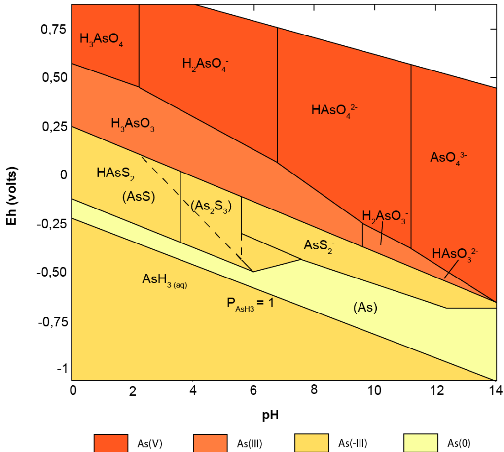
Figure Intr. 1 : Diagramme Eh-pH de l'arsenic (Wang and Mulligan, 2006) à 25°C, 101.3 kPa avec une concentration en As de 10^{-5} mol L -1 et une concentration en soufre de 10^{-3} mol L -1
