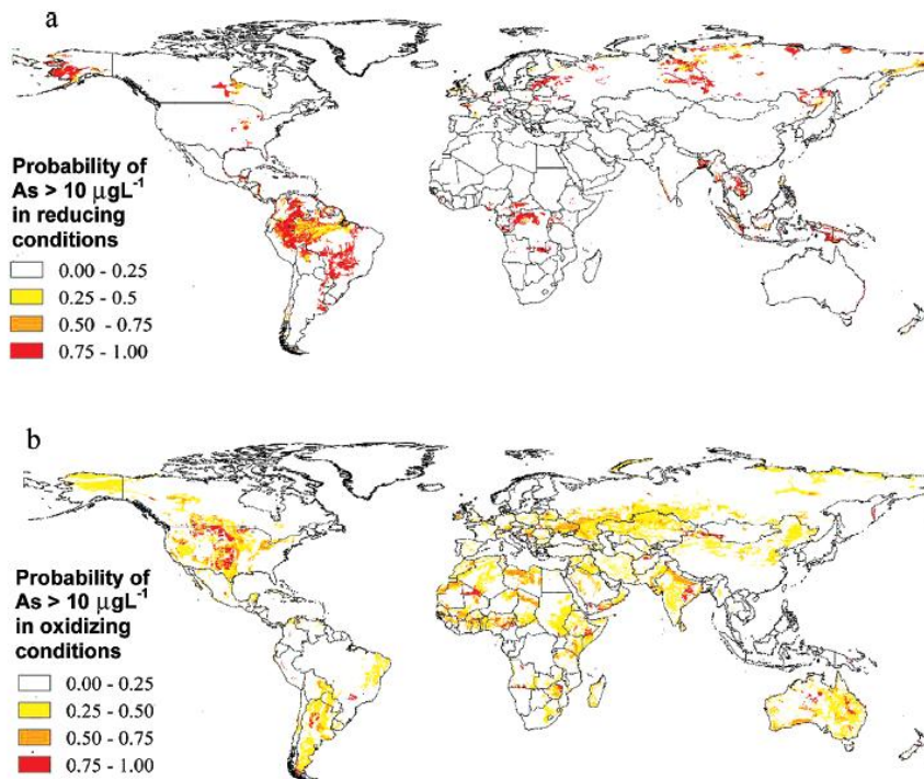
Figure Intr. 3 : Carte de probabilité de contamination en As dans les eaux souterraines a - en conditions réductrices et b - en conditions oxydantes (Amini et al., 2008)
