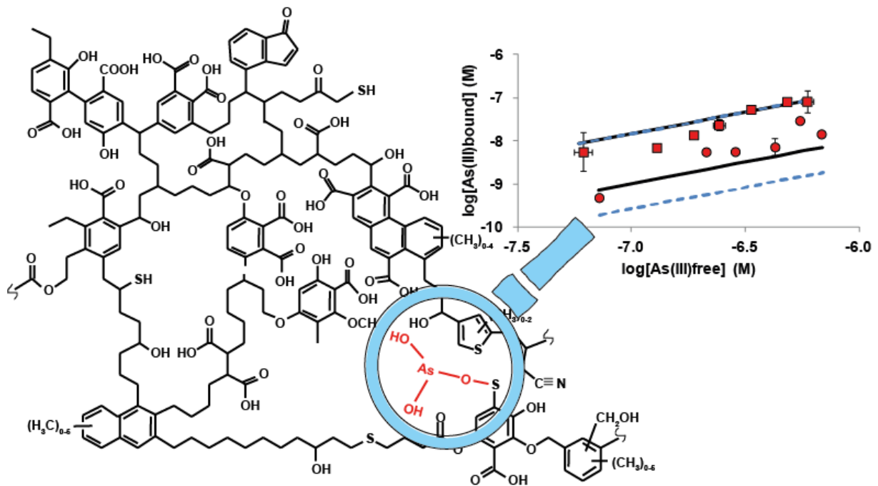
Complexation de l'As(III) par les sites thiols de la matière organique - As(III) complexation through thiol groups of organic matter
