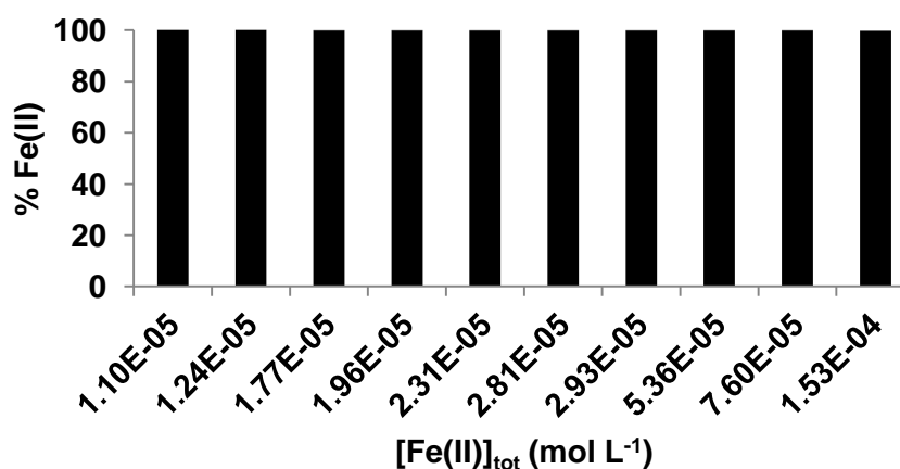
(c) Fe 2+ Fe(OH) +
