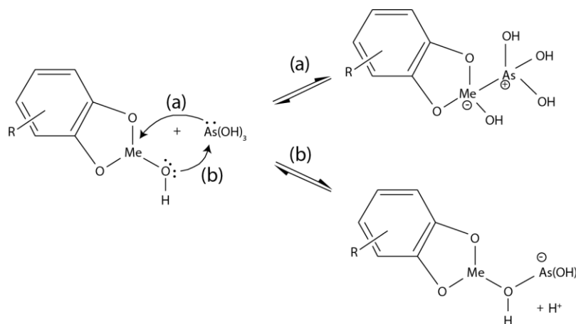
Figure Intr. 9 : Exemple de complexes ternaires entre l'As(III, V), un métal Me et la matière organique (Buschmann et al., 2006)
