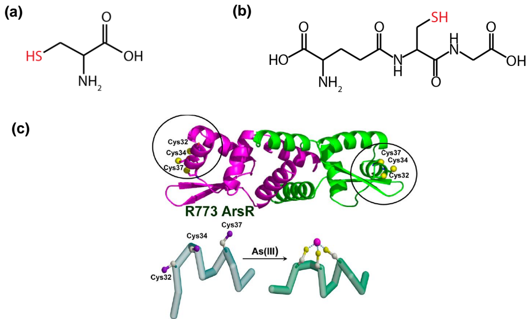
Figure Intr. 4 : Représentations de (a) la cystéine et (b) du glutathion. Les sites thiols sont représentés en rouge. (c) Changements conformationnels après complexation de l'As(III) sur les sites thiols des cystéines de la protéine ArsR de E. coli (Shen et al., 2013)
