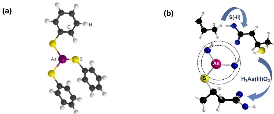
Figure Intr. 8 : Complexation de l'As(III) par (a) trois groupements thiols dans la matière organique et (b) un groupement thiol (Hoffmann et al., 2012; Langner et al., 2011a)
