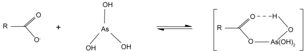
Figure Intr. 7 : Complexation de l'As(III) sur les groupements carboxyliques de la matière organique (Buschmann et al., 2006)
