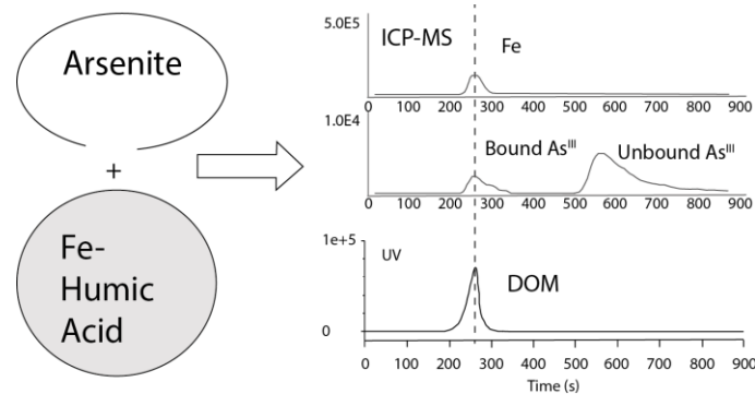
Figure Intr. 10 : Sortie concomitante de l'As(III), du Fe(III) et de la matière organique en sortie de colonne SEC-UV-ICP-MS attestant de la formation de complexes ternaires
