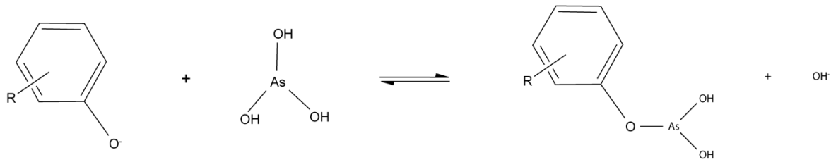
Figure Intr. 6 : Complexation de l'As(III) sur les groupements phénoliques de la matière organique (Buschmann et al., 2006)
