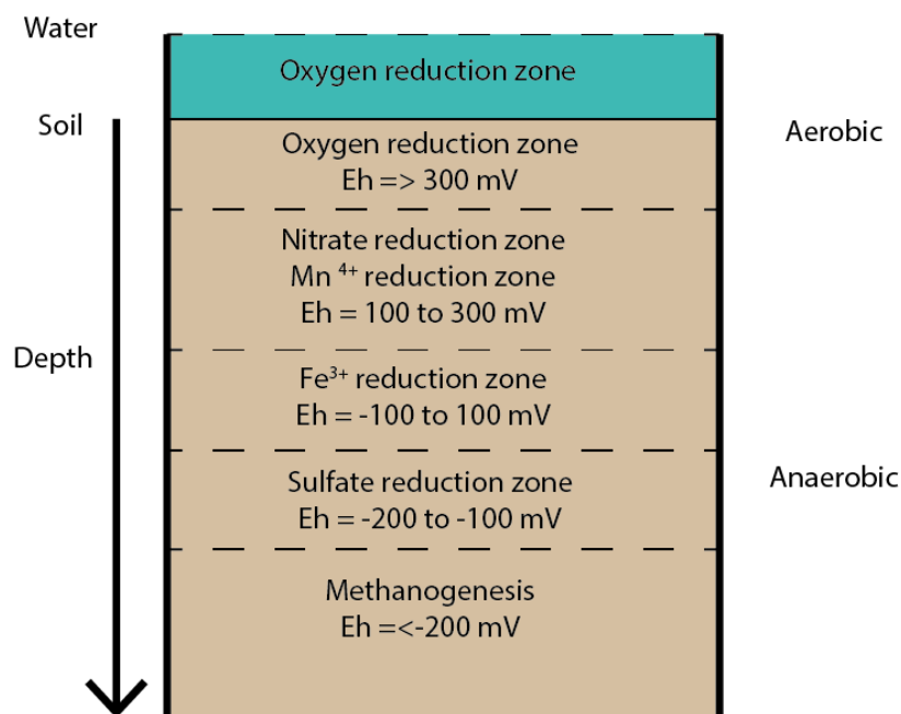
Figure Concl 1 : Distribution verticale de la gamme des espèces électrons accepteurs dans le sol d'une zone humide (Reddy and DeLaune, 2008)
