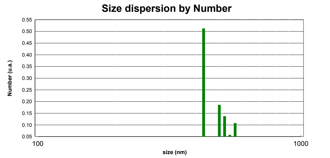
Figure 2 - résultats d'analyse par DLS d'un échantillon de NPs d'hématite synthétisée.
