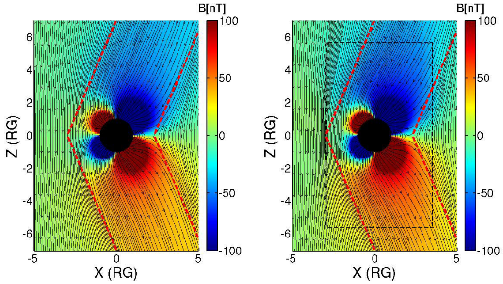
FIGURE 5.1 – Les couleurs représentent la composante B_x du champ magnétique dans le plan XZ pour la simulation 1 à gauche et la simulation 2 à droite. Les lignes noires représentent les lignes de champ magnétiques simulées et les traits pointillés rouges montrent l'emplacement théorique des ailes d'Alfvén. Sur la figure de droite, les limites de la région mieux résolue sont représentées par les traits pointillés noirs.
