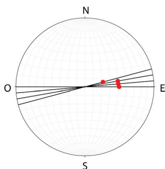
Figure 5-18 : Stéréogramme des plans de charnières (en noir) et d'azimuts des axes (en rouge) des plis isoclinaux décrits au Nord-Est de Trevillach.
