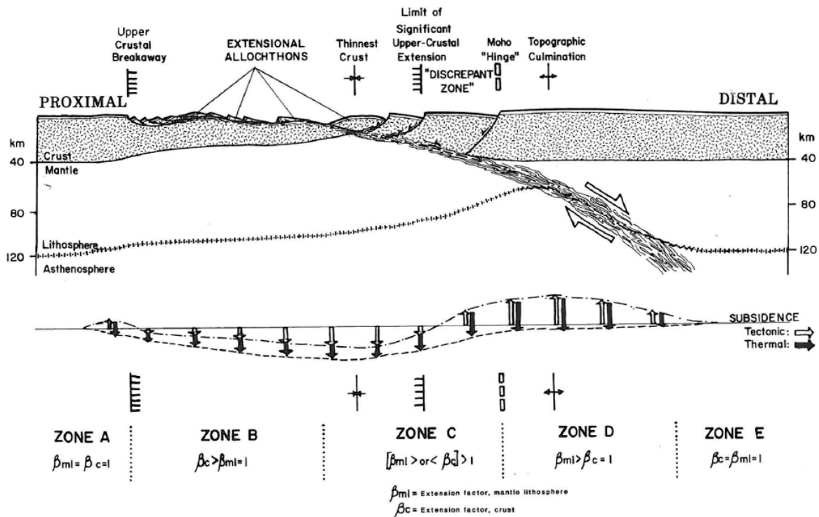
Figure 1-4 : Modèle de rift en cisaillement simple (Wernicke, 1985).
