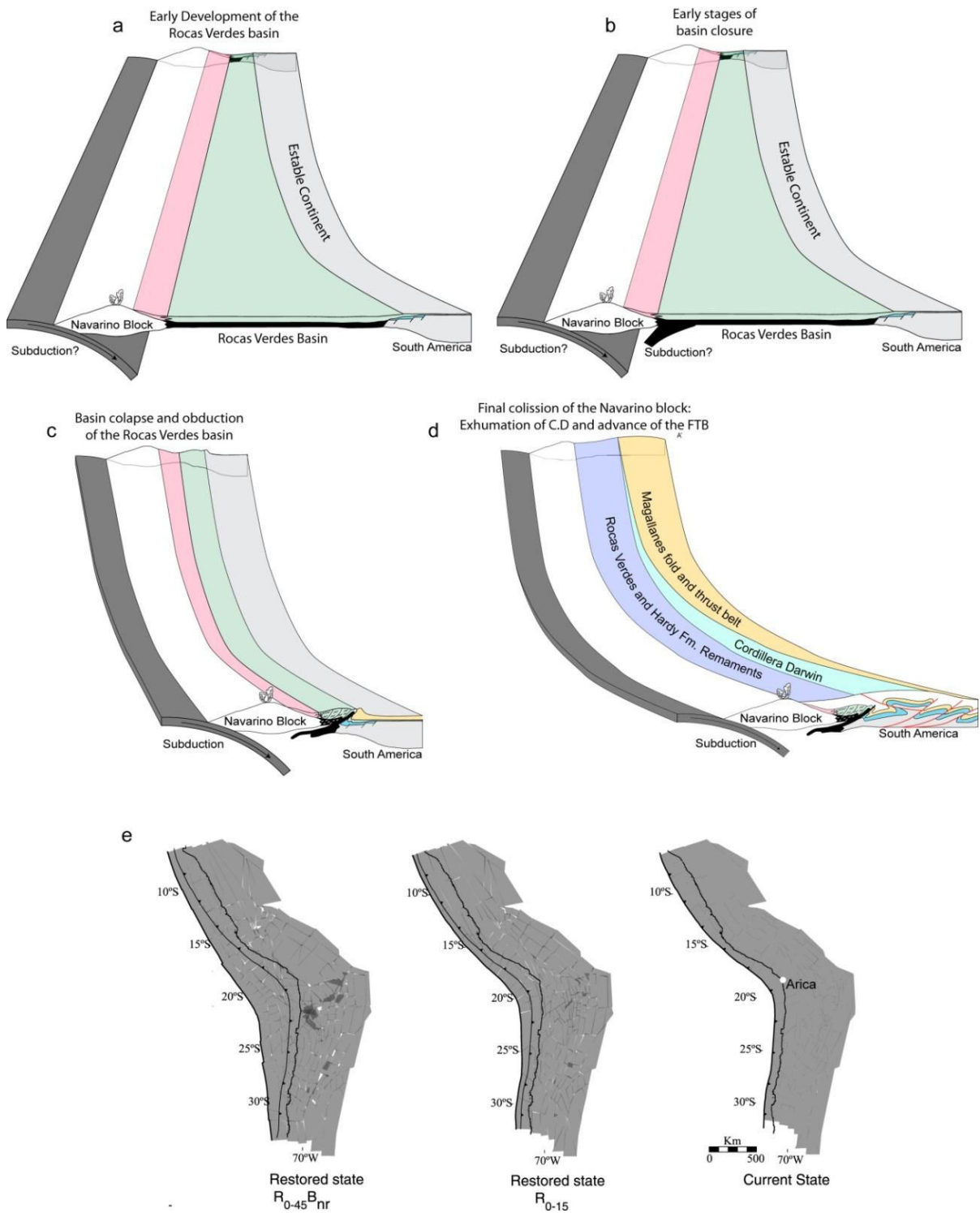
Figura 5.3.1: Modelo esquemático de la evolución de los Andes Fueguinas (a-d) y del Oroclino Boliviano (modificado de Arriagada et al. (2008) ) (e). Los perfiles en a-d son modificados de ( Klepeis et al., 2010 ).
