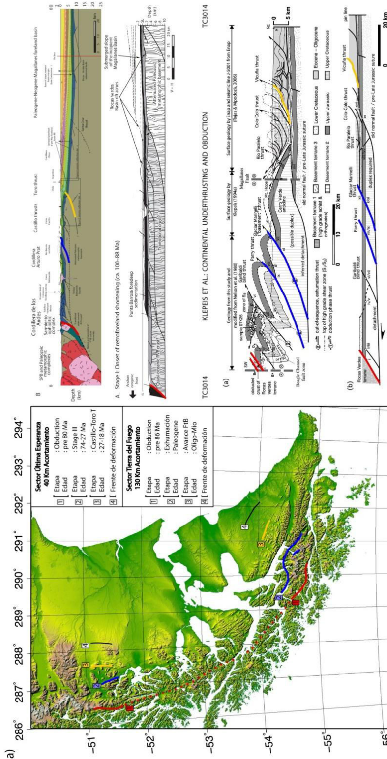
Figura 1.3.3: a) Ubicación en plantas de las estructuras seleccionadas en los perfiles b (Fosdick et al., 2011) y c (Klepeis et al., 2010). Línea roja corresponde a la estructura que participa en los procesos de obducción de las Rocas Verdes; línea roja es la conexión inferida entre ambas regiones. En azul estructuras que participan en los procesos de exhumación. En el sector de Última Esperanza esta estructura es la Falla Tenerife, mientras que en el sector de Cordillera Darwin se han reconocido al menos tres fallas que participan en los procesos de exhumación, falla Garibaldi (no mostrada en el mapa), falla Parry y la falla Glaciar Marinelli. b y c) Perfiles y secciones restauradas donde se observan los diferentes estilos estructurales (modificado de Fosdick et al. (2011) y Klepeis et al. (2010)). El acortamiento calculado en ambos perfiles es entre 1 y 3 y no consideran en el acortamiento relacionado a la obducción de las Rocas Verdes
