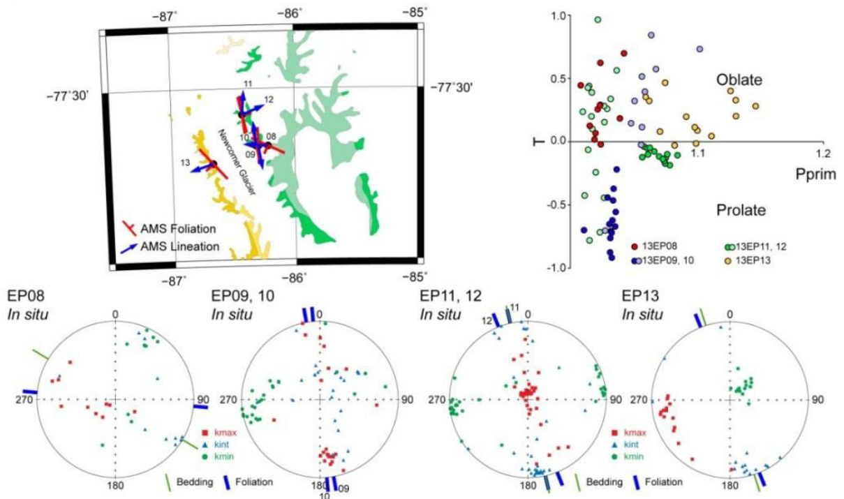
Figura A1.5: Ubicación y resultados de la anisotropía de susceptibilidad magnética. a) Cordón Heritage: 1, ubicación de los sitios mostrando la lineación y foliación magnética (ver Fig. 2 para ubicación general y leyenda); 2, Diagramas T-P; 3, Proyecciones de áreas equivalentes de los elipsoides de la AMS para cada muestra (líneas verdes indican la dirección del rumbo de las capas y las líneas azules la foliación). b) Cordón Sentinel. Misma simbología que en a).
