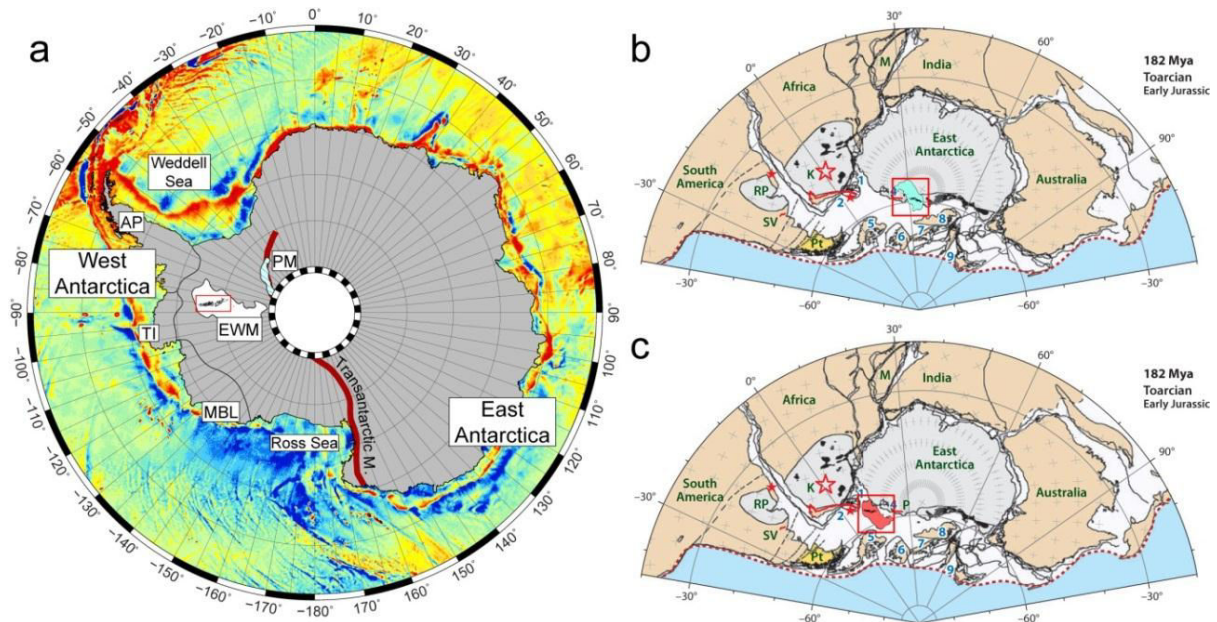
Figura A1.1: a) Antártica. b y c) modelos de la posición de los Montes Ellsworth anterior al quiebre de Gondwana. La figura base está tomada de Dalziel et al., 2013 ; b: modelo tomado de Schmidt y Rowley, 1986 ; c: modelo de Dalziel et al., 2013 . AP, Antarctic Peninsula; TI, Turston Island; MBL Marie Byrd Land; EWM, Ellsworth-Withmoure mountains; PM, Pensacola Mountains.
