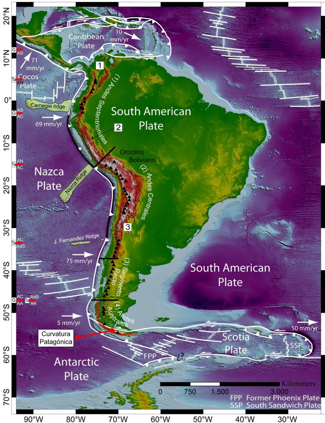
Figure F.1: Cordillère des Andes: contexte général. Les segments noirs dans la zone de subduction correspondent à une subduction plane. G/Ta sont les subdivisions proposées par Gansser (1973)/Tassara et Yañez (2010) , pour lesquelles: AS: Andes Septentrionales; AN: Andes du Nord; AC: Andes Centrales; AdS: Andes du Sud; AA: Andes Australes. Triangles (Nord, Centre Sud, Austral); 1, 2 et 3 sont les écarts volcaniques. Modifié après ( Barker, 2001 ; Gansser, 1973 ; Jordan et al., 1983 ; Mann et al., 2002 ; Ramos, 2009 ; Smalley et al., 2007 ; Trenkamp et al., 2002 ).
