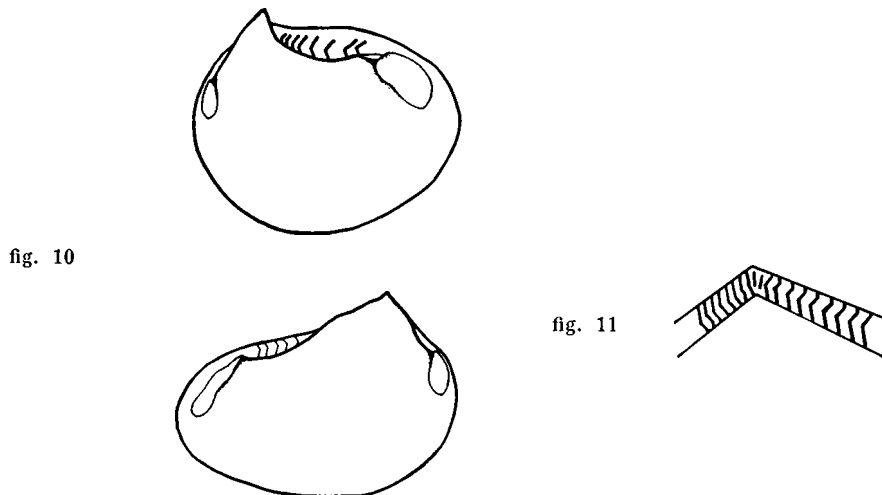
Fig. 10 et 11. — Ctenodonta ciae
