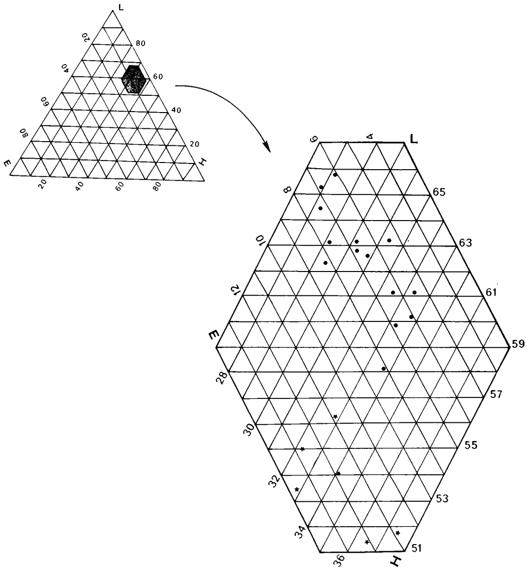
Fig. 44. — Comparaison de N. subrectangularis (·) BABIN 1963 et de N. septulatus (*) nov. sp. en coordonnées triangulaires pour les variables L, h, e. Le diagramme de gauche montre la position de la partie grossie à droite (explications p. 22).
