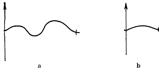
Fig. 91. — Tornoceras simplex : exemplaires du Frasnien de Rostellec a - suture d'un adulte b - suture d'un très jeune individu
