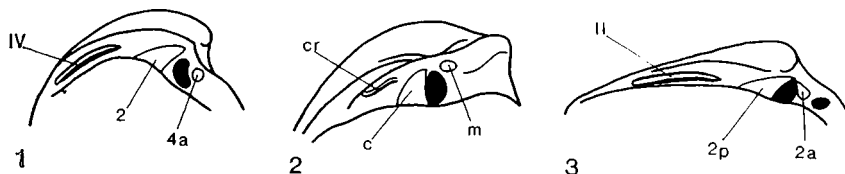
Fig. 74. — 1 - Megalodon (d'après HAFFER). 2 - Goniophora (d'après RUZICKA & PRANTL) : cr = « crête sur plateau cardinal » (= vestige d'une dent latérale ?). 3 - Mecynodon (d'après HAFFER).
