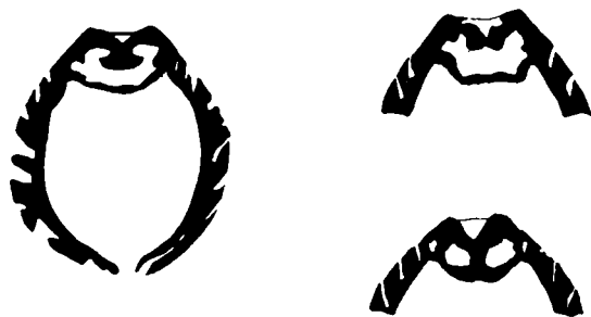
Fig. 55. — Coupes transversales de Conocardium artifex effectuées à partir de l'extrémité antérieure en allant vers l'umbo ; la coupe de gauche montre l'ensemble à 4 mm du crochet environ ; les 2 autres représentent seulement la partie supérieure de la section à 2,5 et à 0,5 mm du crochet.
