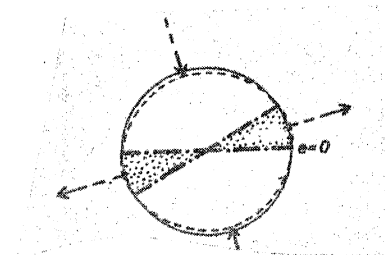
Déformation infinitésimale
