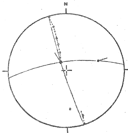
Fig. 60 : Exemple de trajet de dispersion de la linéation Lel intermédiaire entre un grand cercle et un petit cercle (La pointe du Puits).
