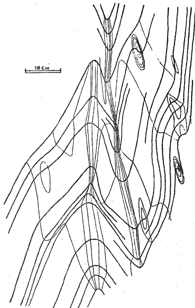
Fig. 58 : Courbe t'\alpha/\alpha - Plis P2 affectant un niveau calco-silicaté (en grisé) - Anse de La Gauthier.
