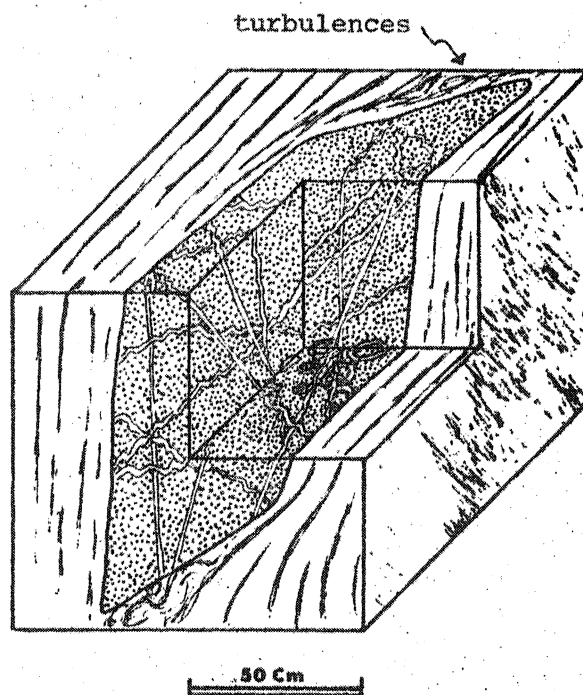
Fig. 100 : Bloc diagramme montrant les relations géométriques existant entre la forme et les positions des enclaves sub-rhombéoédriques de gneiss à grain fin et le rubanement des gneiss granitoïdes. On note l'existence de veines plissées sur deux axes (structures en dômes et bassins) et l'absence de veines boudinées dans l'enclave.
