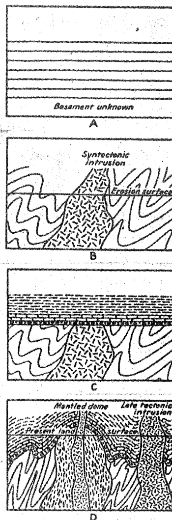
Fig. 102 : L'origine des mantled gneiss domes d'après ESKOLA (1949).
