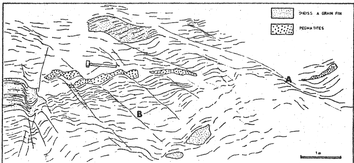
Fig.22 RESEAU DE CISAILEMENTS DANS LES GNEISS GRANITOIDES RUBANNES DE LA DAME JOUANNE - ST BRIAC
