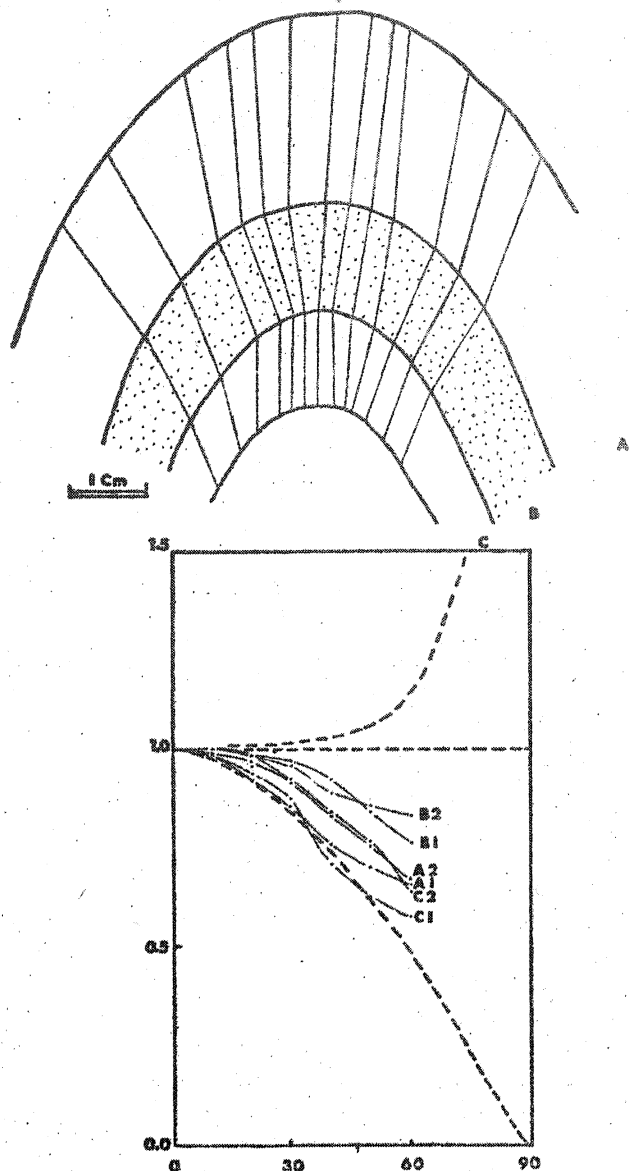
Fig. 82 : Courbes t'\alpha/\alpha - Pli P3 affectant un niveau calco-silicaté (en grisé) dans les gneiss à grain fin de l'anse de La Gauthier.
