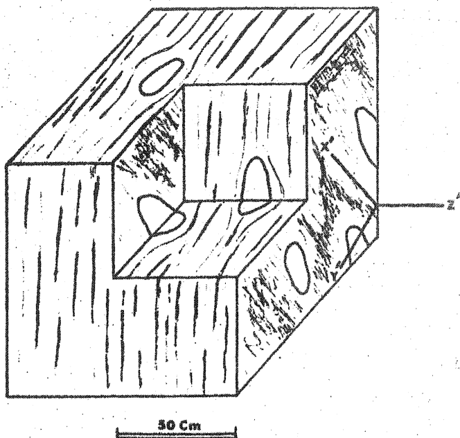
Fig. 97 : Bloc diagramme montrant les caractéristiques géométriques des gneiss granitoïdes rubanés. Le plan de rubanement détermine le plan X'Y' , et l'orientation préférentielle du grand axe des enclaves l'axe X' .
