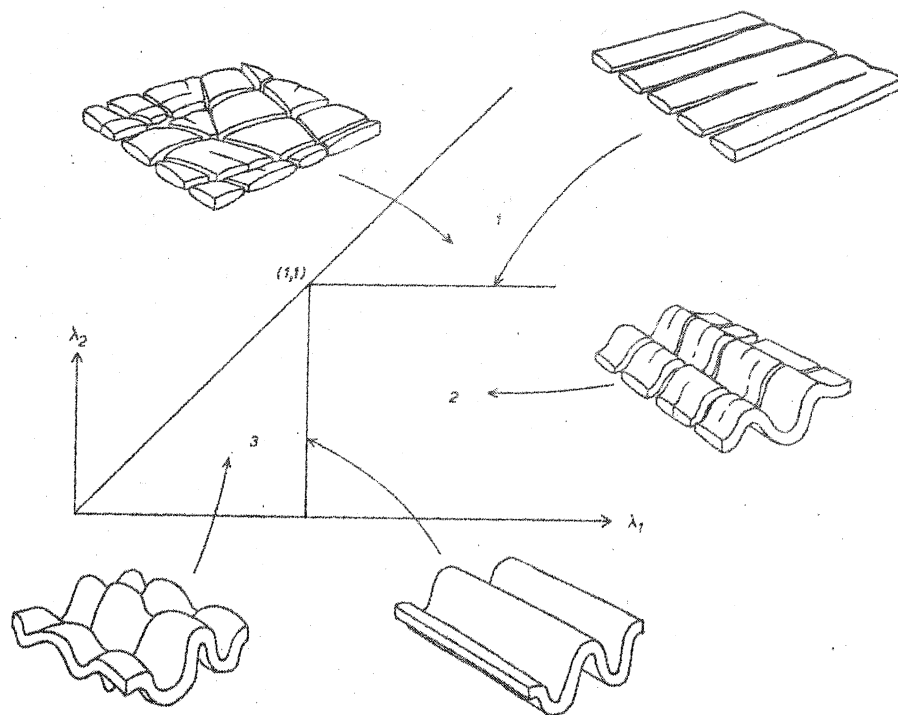
Fig. 38 : Représentation des cinq types de structures, pouvant affecter une veine minérale, en fonction du type de l'ellipse de déformation (voir fig. 29).
