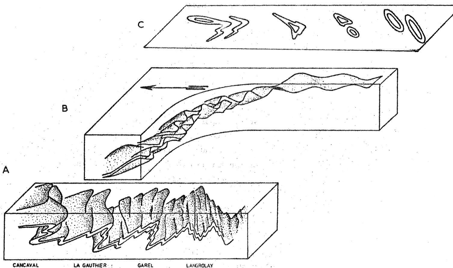
Fig. 12 : Schémas résumant, de Langrolay à Cancaval, l'évolution des plis P2 (A), des plis P3 (B) et de leurs interférences dans un plan horizontal (C).
