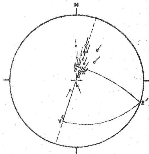
Fig. 98 : Exemple de détermination du système d'axes principaux X' , Y' , Z' dans les gneiss granitoïdes rubanés de la Promenade au Clair de Lune.
