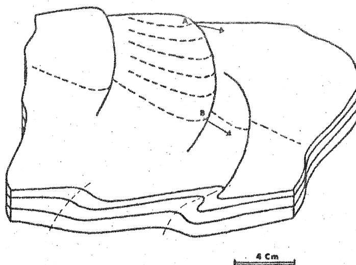
Fig. 71 : Pli P2 en gousse déformant la linéation précoce Lé2. Les lignes de glissement (flèches) sont légèrement dispersées (comparer avec la fig. 69) et font avec l'axe du pli un angle variable décroissant de B en A.
