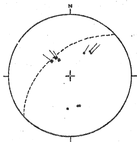
Fig. 62 : Lignes et plans de glissement des plis P2 à La Landriais.
