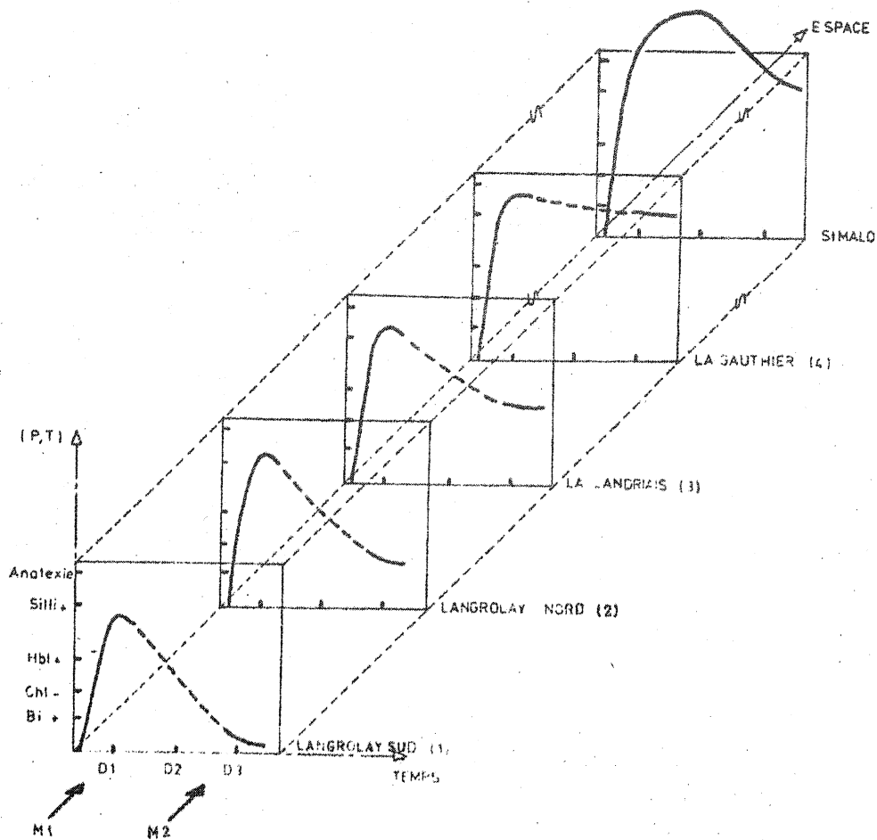
Fig. 25 : Schémas montrant l'évolution spatio-temporelle des conditions de métamorphisme le long de la Vallée de la Rance (cf. Fig. 24).
