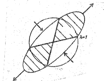
Déformation finie
