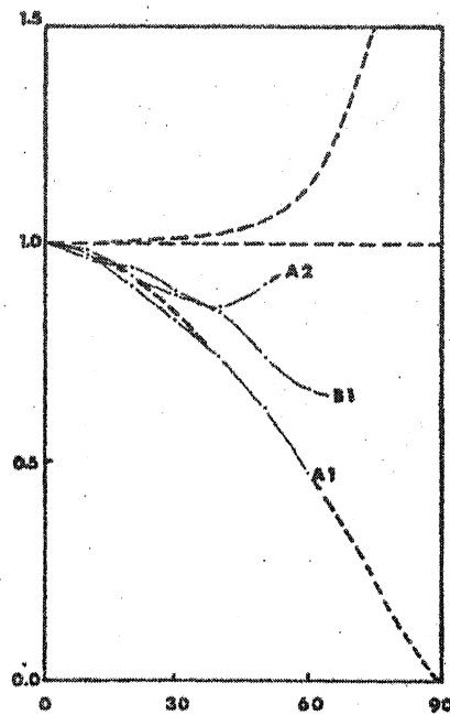
Fig. 54 : Courbes t'\alpha/\alpha - Plis P2 asymétrique dans les gneiss à grain fin de La Landriais. 1- flanc court 2- flanc long.
