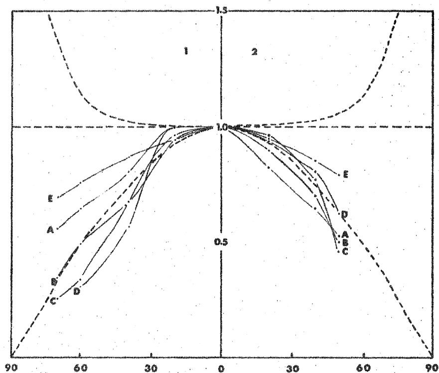
Fig. 73 : Courbes t'\alpha/\alpha - Pli P2 dans les gneiss à grain fin de Cancaval.
