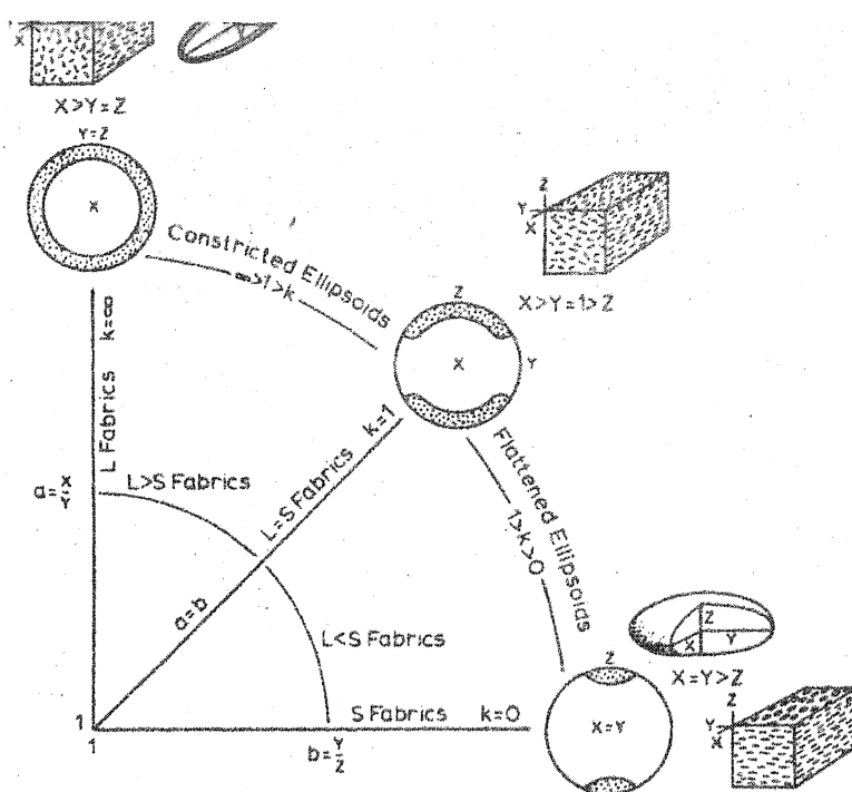
Fig. 37 : Diagramme de PLINN, montrant les relations entre les fabriques L-S et l'ellipsoïde de déformation. Les stéréogrammes montrent la répartition des pôles des minéraux planaires représentés sur les blocs diagrammes.
