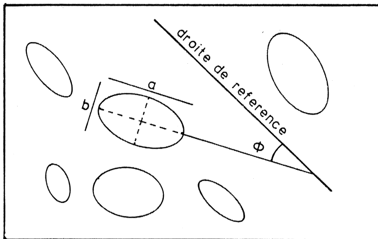
Fig. 7 - Technique de mesure des marqueurs elliptiques.
