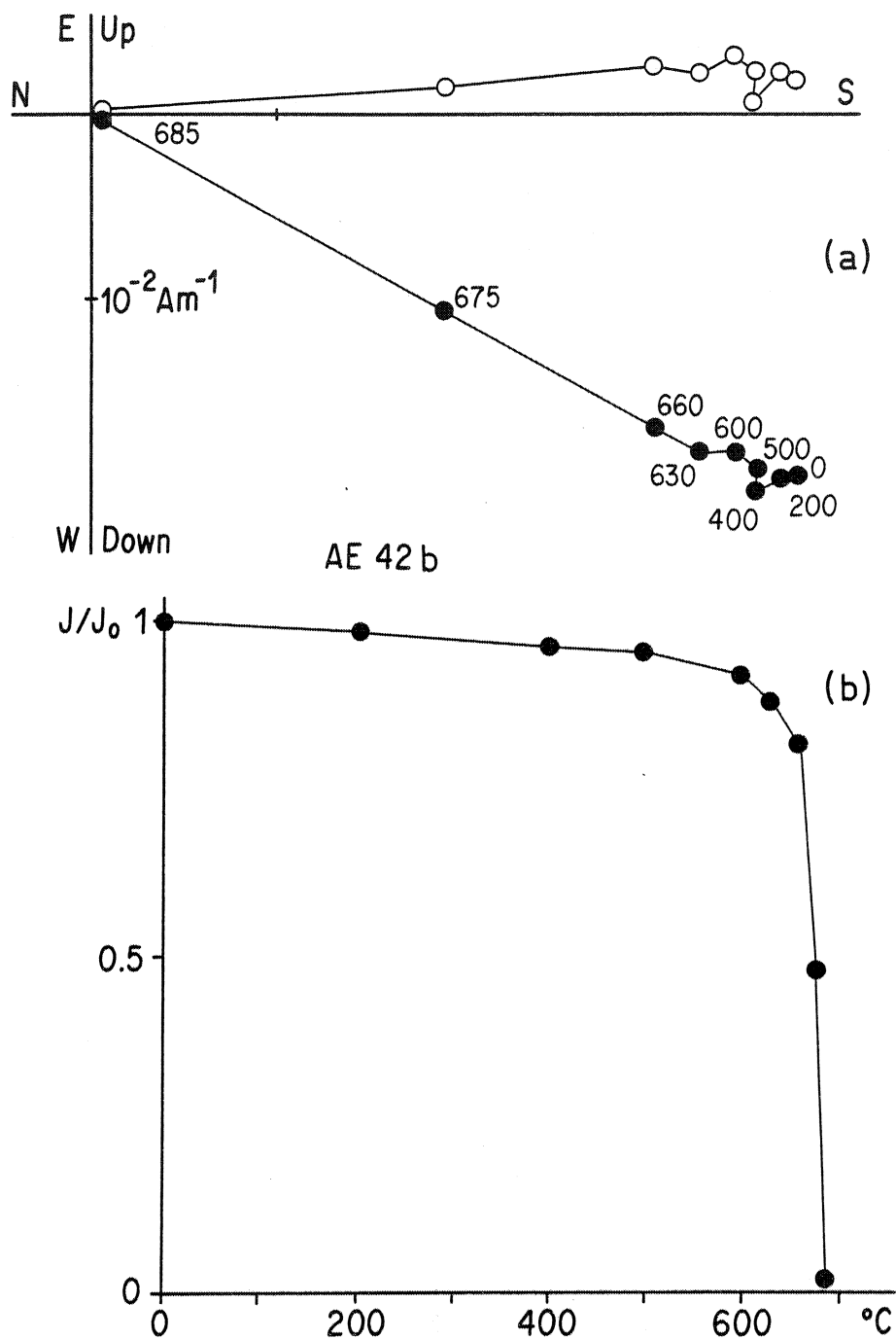
Fig. 25 - Désaimantation thermique d'un échantillon du site E. (a) diagramme de Zijderveld ; les chiffres sur la courbe indiquent les températures en °C. (b) Evolution de l'intensité en fonction de la température.
