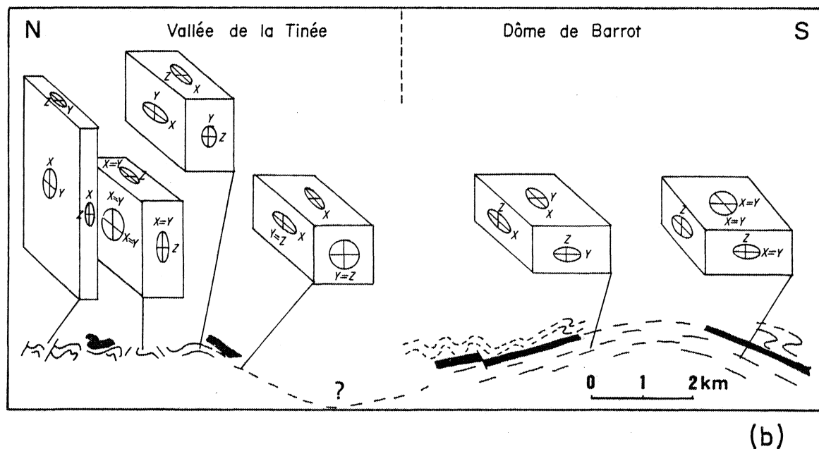
Fig. 13 - Les séries rouges permienes des Alpes Maritimes (a) : principaux affleurements (b) coupeschématique, du Sud au Nord, du Dôme de Barrot et de la Vallée de la Tinée ; les blocs-diagrammes illustrent les différents stades de déformation croissante (d'après Graham, 1978a).
