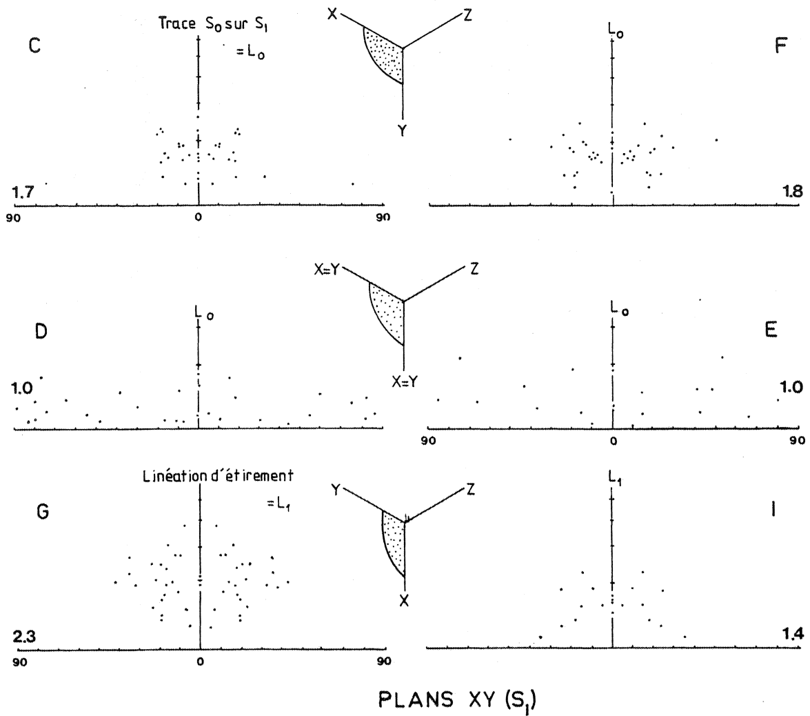
Fig. 17 - Vallée de la Tinée : diagrammes Rf/\phi des mesures effectuées dans le plan de schistosité. Les systèmes d'axes XYZ illustrent de manière schématique l'évolution des axes de la déformation entre les sites ; pointillé : plan de mesure. Les rapports moyens déterminés sont reportés sur ces diagrammes.
