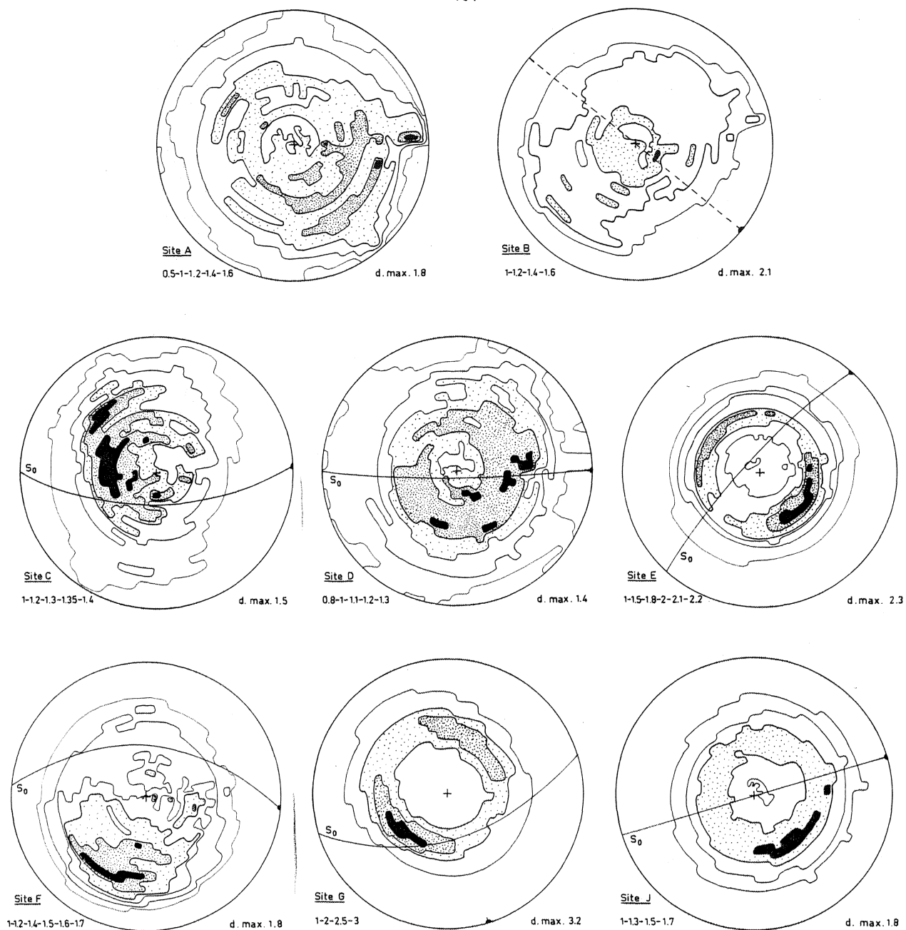
Fig. 87 - Orientations préférentielles des axes \langle 104 \rangle de l'hématite dans les échantillons des Alpes Maritimes. Projection stéréographique dans l'hémisphère supérieur. Densité maximum (d. max.) et contours indiqués en multiples d'une distribution uniforme. Plans d'exploration : Sites A et B : S_0 ; Sites C à G : S_1 .
