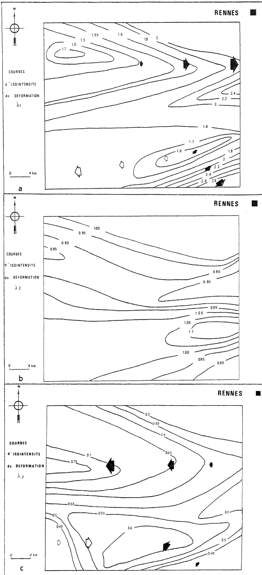
Fig. 15 - Courbes d'intensité de déformation obtenues par interpolation linéaire entre les points.
