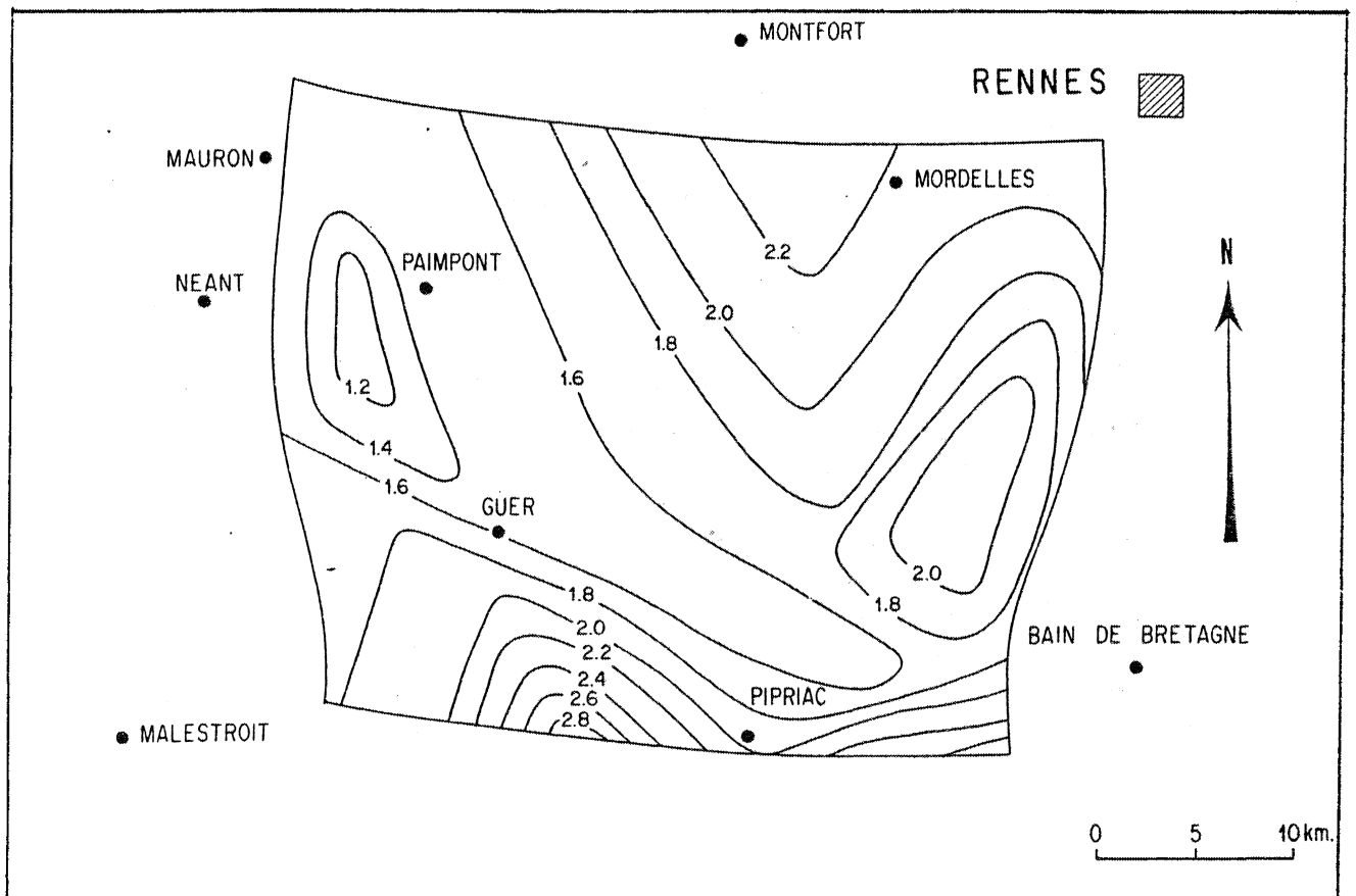
Fig. 11 - Carte des contours d'isointensité de l'étirement principal \lambda_2 obtenus par interpolation graphique des données du tableau 7 (colonne 6).
