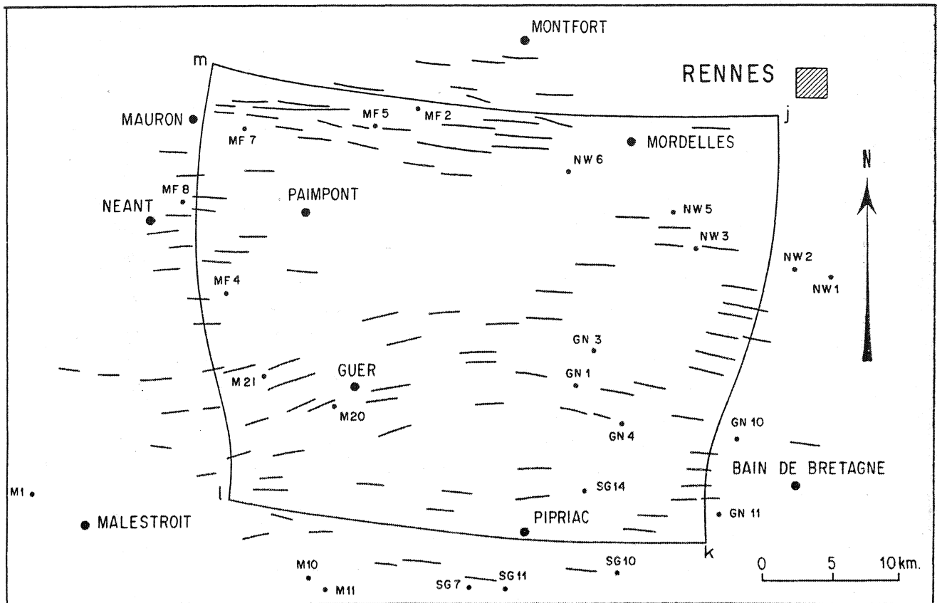
Fig. 10 - Données de mesures de déformation sur la région. Lignes fines - traces de schistosité NW2, NW3 - localisation des mesures jklm - domaine considéré pour la déformation inverse
