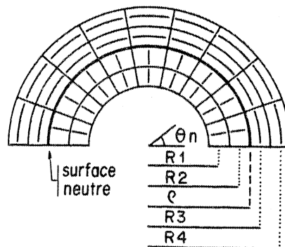
Fig. 12 - b .trace de la schistosité dans chaque élément du pli.
