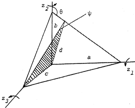
Fig. 7 - Représentation d'un plan d'azimut \theta et de pendage \psi d'équation az_1 + bz_2 + cz_3 + d = 0
