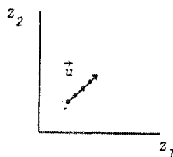
Fig. 10 - Représentation du vecteur \vec{u} en n vecteurs élémentaires dans le repère z_1 z_2
