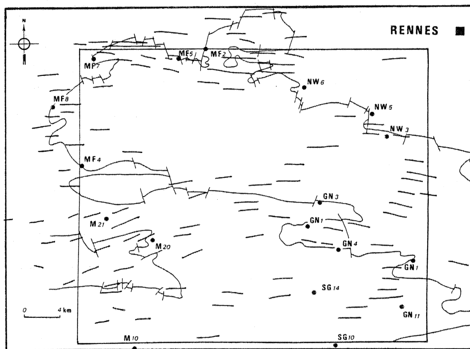
Fig. 16 - Carte des traces du plan principal de schistosité X_1 X_2 (C. Le Corre, 1978) et des sites de mesures de déformation finie (cf. Fig. 6). Le domaine d'étude est limité par le rectangle intérieur. Les traces de schistosité indiquent la projection de l'axe principal de déformation \lambda_1 dans le plan horizontal.
