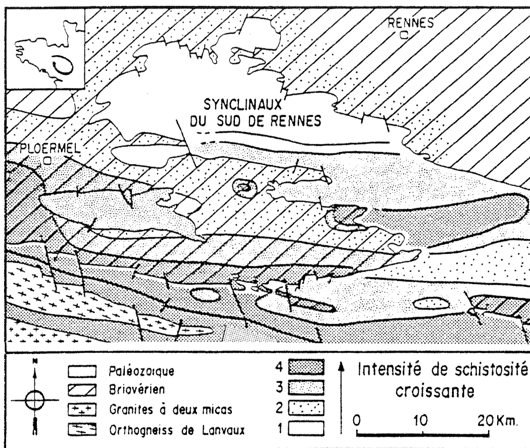
Fig. 5 - Carte des variations de typologie de la schistosité dans la région étudiée. D'après C. Le Corre (1978).
