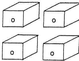
Fig.C9 - a : réseau d'éléments finis : les éléments de bordure n'interviennent pas dans le calcul de SUM
