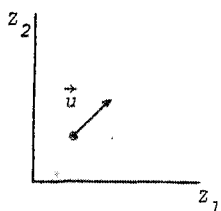
Fig. 9 - Représentation du vecteur \vec{u} dans le repère z_1 z_2
