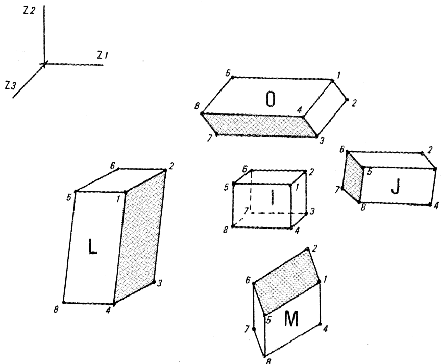
Fig. A3 - L'élément central I est entouré par 4 voisins immédiats, J , O , L , M . Les coins des éléments sont indiqués de 1 à 8.
