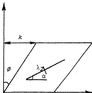
Fig. 14 - Déformation d'un élément rectangulaire k taux de cisaillement \phi angle de cisaillement \alpha orientation de l'axe principal de déformation \lambda_1 . \lambda_1 \lambda_2 axes principaux de déformation
