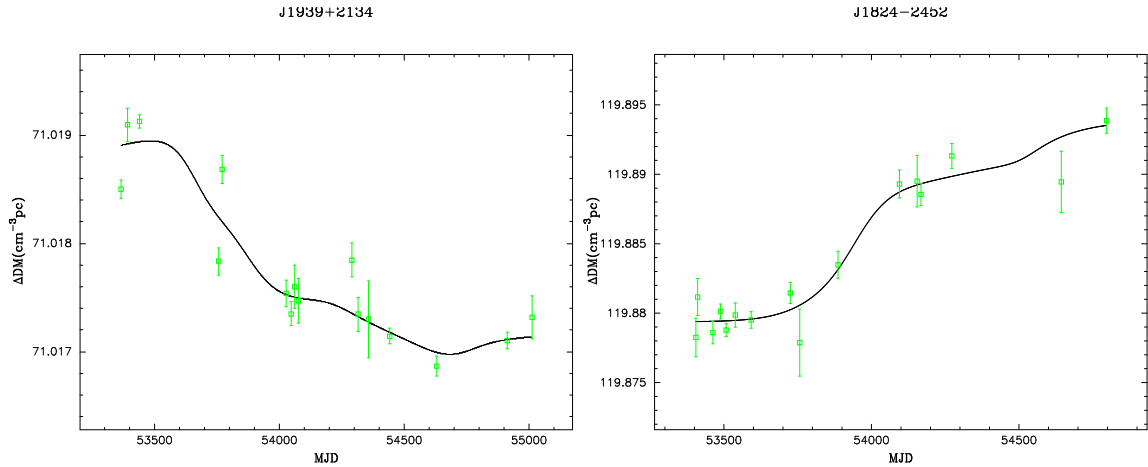
FIGURE 5.1: Variation de la mesure de dispersion des pulsars J1939+2134 et J1824-2452. Ces graphiques ont été obtenus avec TEMP02 et le plugin calcDMe . Les points ont été obtenus à des époques où des observations à deux fréquences sont disponibles. La courbe lisse les variations sur 130 jours.
