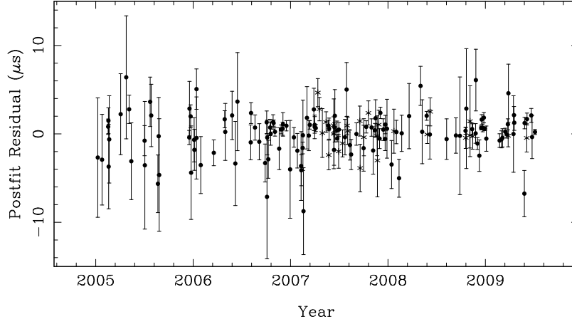
FIGURE 5.21: Résidus de chronométrage de J2145-0750.
